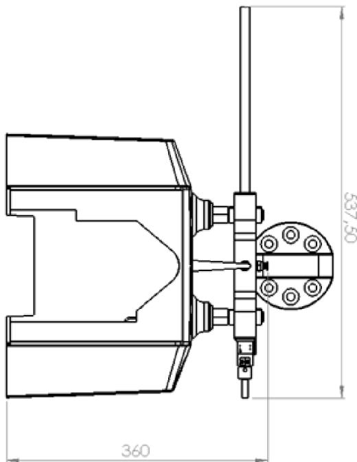
Obr. 44 Varianta A – hlavní rozměry
