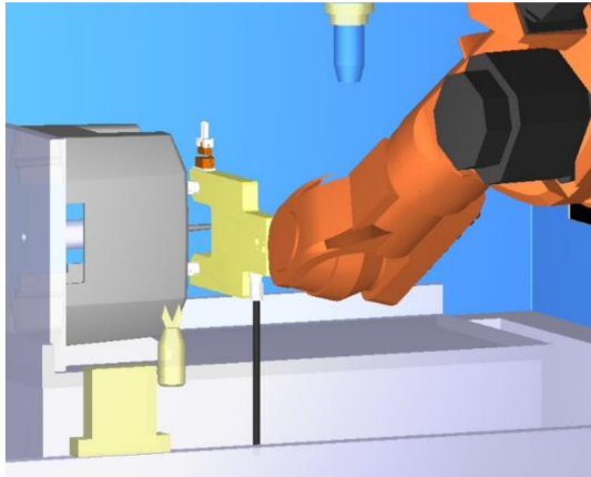
Obr. 70 Vložení do aretačního přípravku - RoboDK
