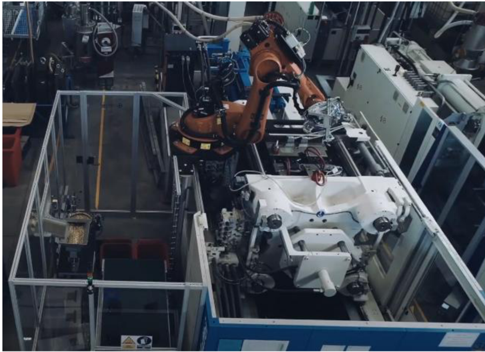
Obr. 23 Robotické pracoviště – Dentec [14]
