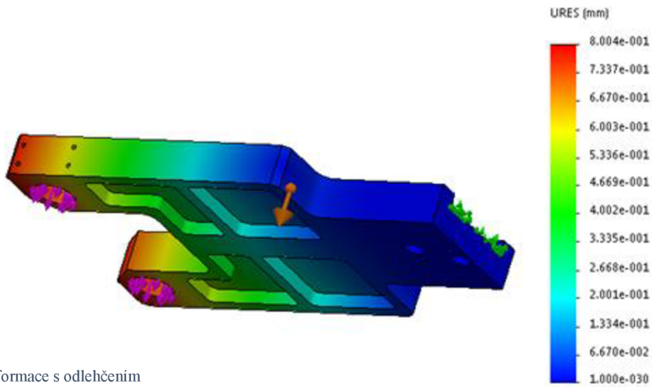
Obr. 49 Deformace-bez odlehčení
