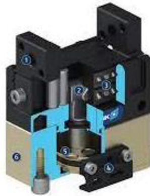
Obr. 59 Chapadla Schunk MPG 25 – řez [21]
