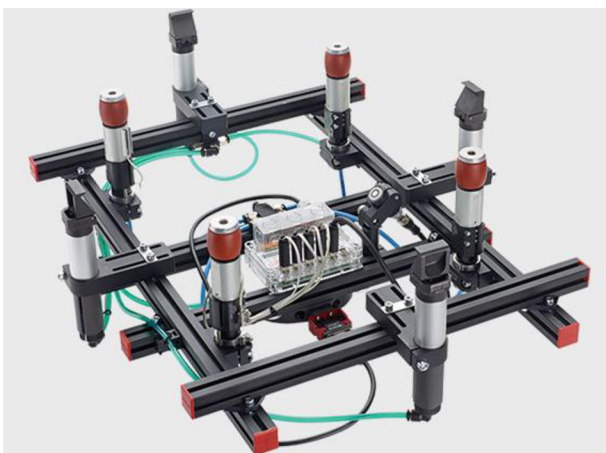
Obr. 5 Modulové efektor [5]
