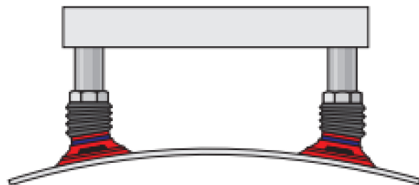
Obr. 12 Kloubový kompenzátor [8]
