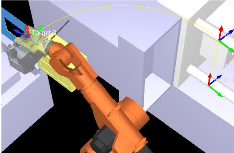
Obr. 55 Pohyb robotu – cílová pozice
