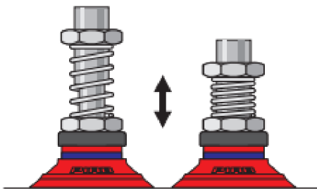
Obr. 11 Výškový kompenzátor [8]
