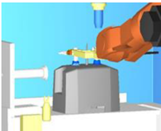
Obr. 72 Zafrezování vtoku - RoboDK
