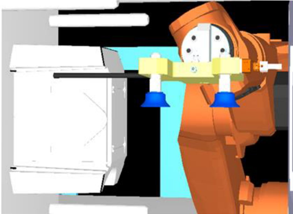
Obr. 65 Vkládání zálišků do dutiny formy - RoboDK
