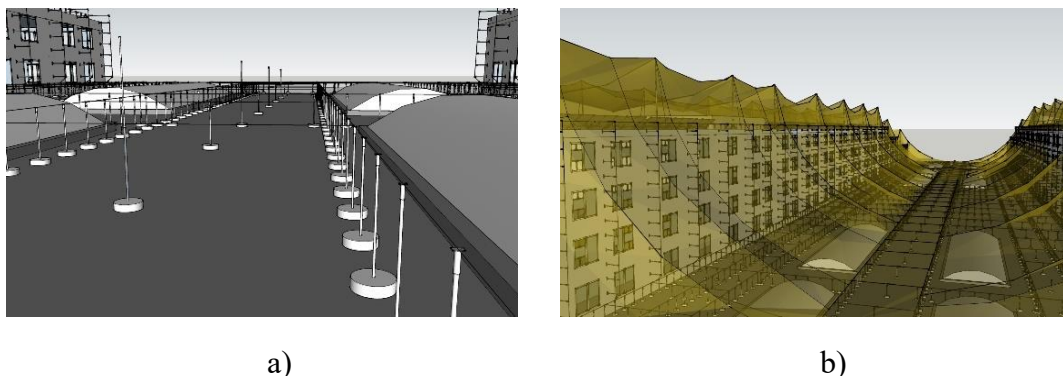
Obrázek 7.24 Ochrana bloku F: a) ochrana světlíků přidáním izolovaných jímacích tyčí, b) ochranný prostor bloku F
