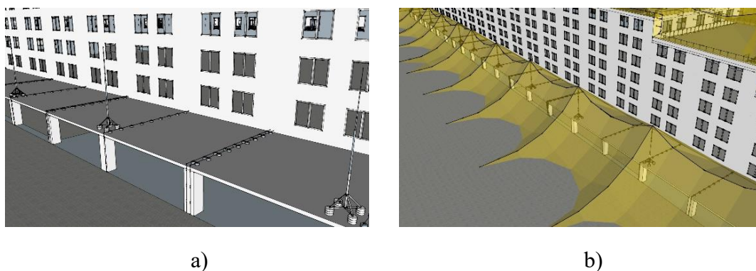
Obrázek 7.25 Ochrana severního a jižního bloku: a) část jímací soustavy na jižním bloku, b) ochrana severního a jižního bloku
