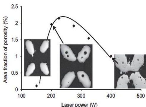
Obr. 2-3 Zmena porozity v závislosti od výkonu lasera. [5]
