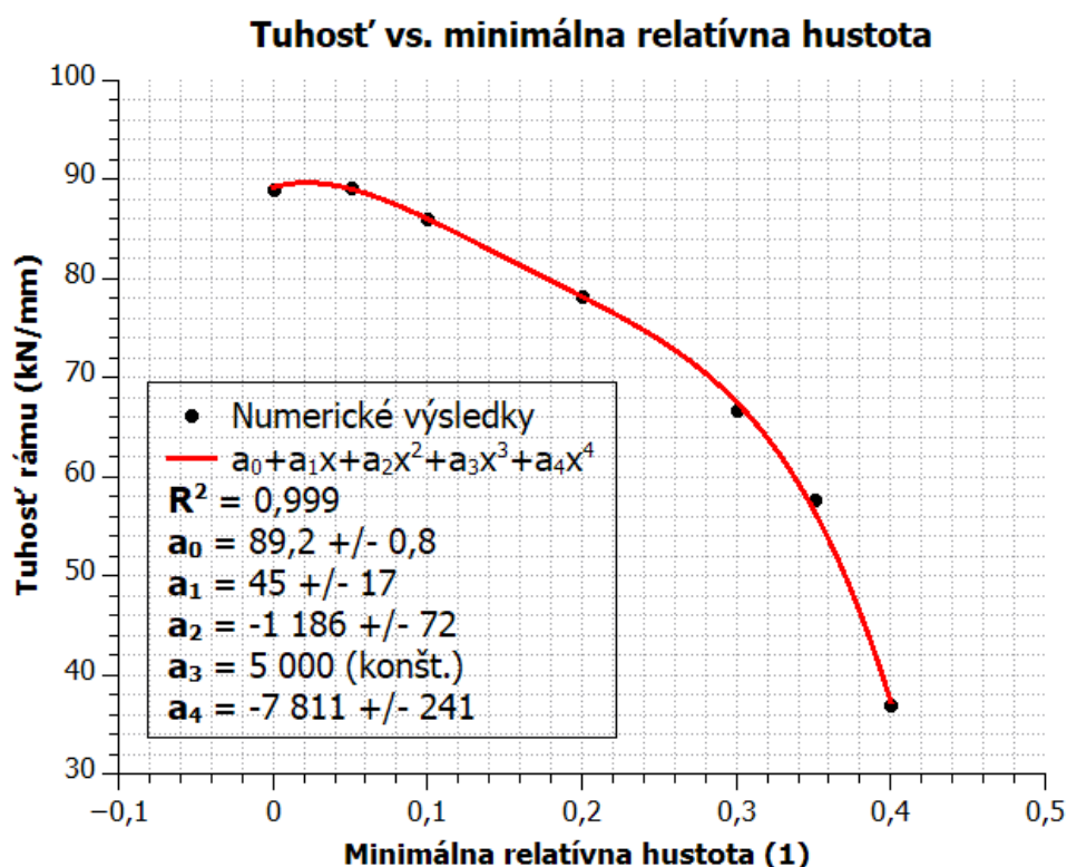
Obr. 5-3 Tuhosť vs. minimálna relatívna hustota.
