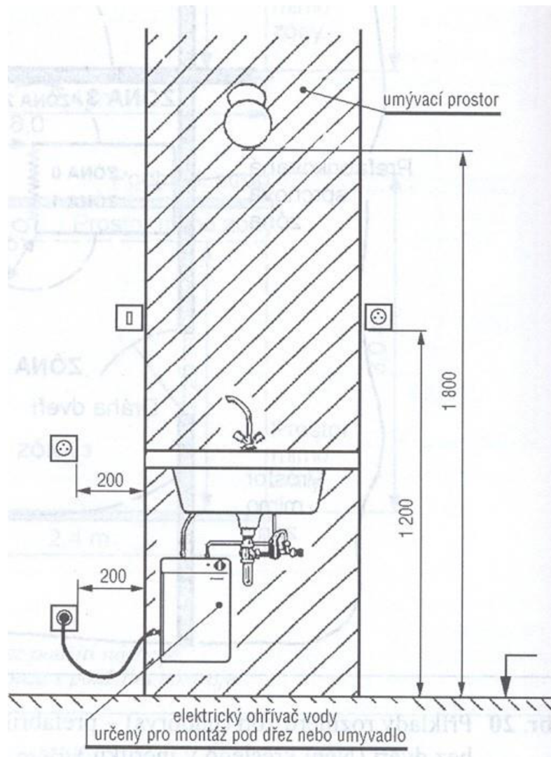
Obr. 12 Umývací prostor [34]
