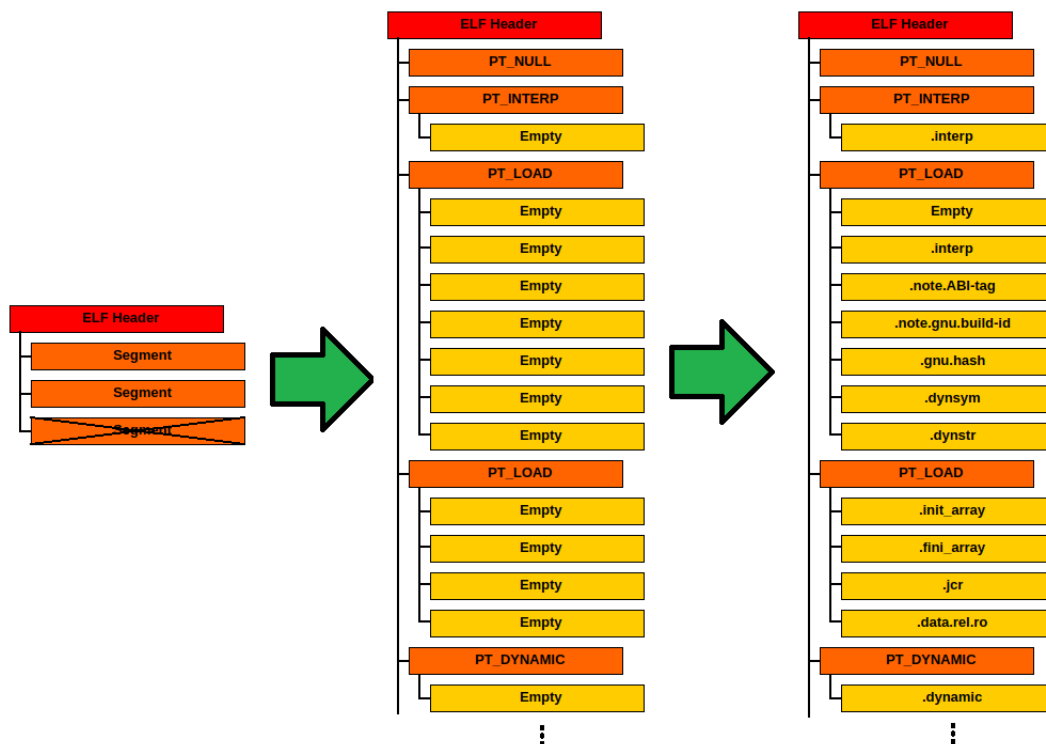
Obrázek 5.4: Jednotlivé kroky úpravy z pohledu grafu sekcí
