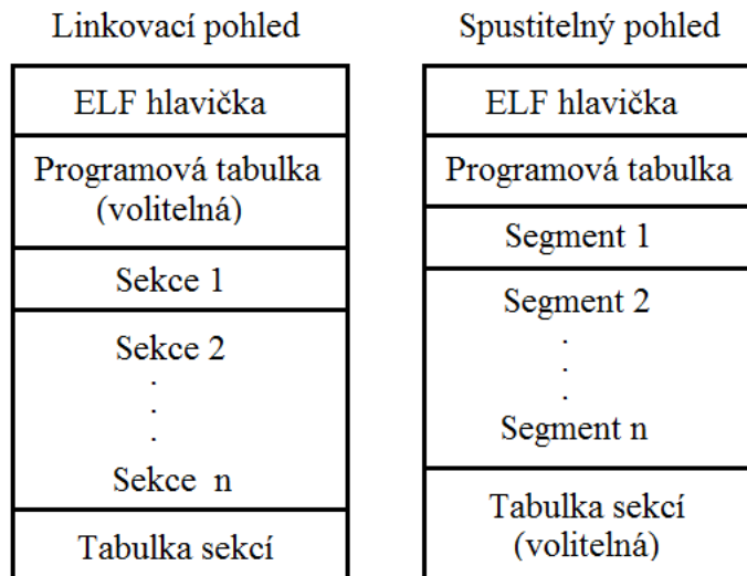
Obrázek 3.1: Formáty objektových souborů [14]
