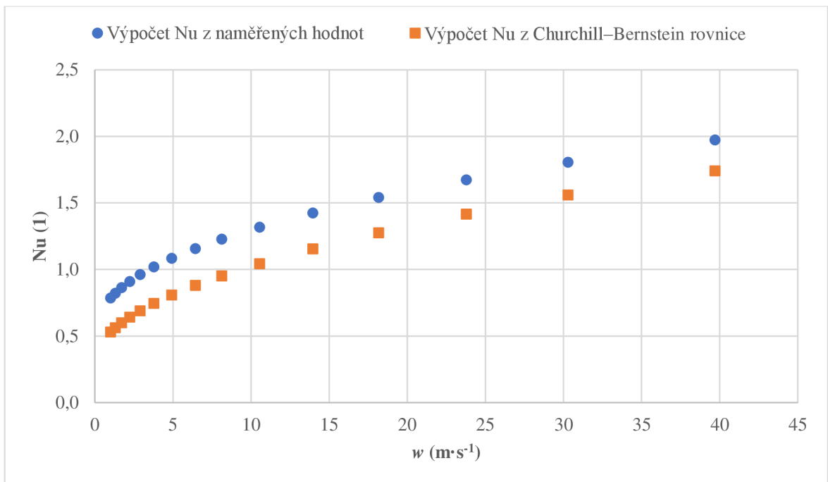
Obr. 4.2.2 Grafická závislost Nusseltova čísla na rychlosti proudění pro \alpha = 0,5
