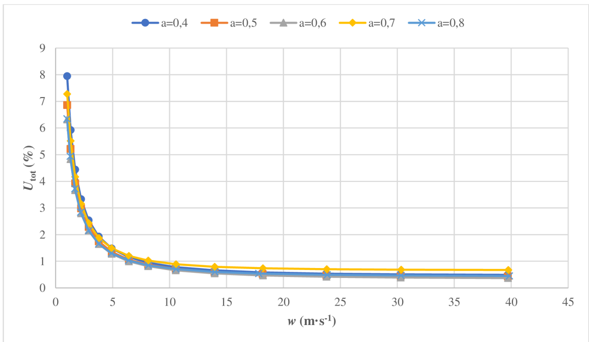
Obr. 3.8 Grafická závislost celkové relativní nejistoty na rychlosti
