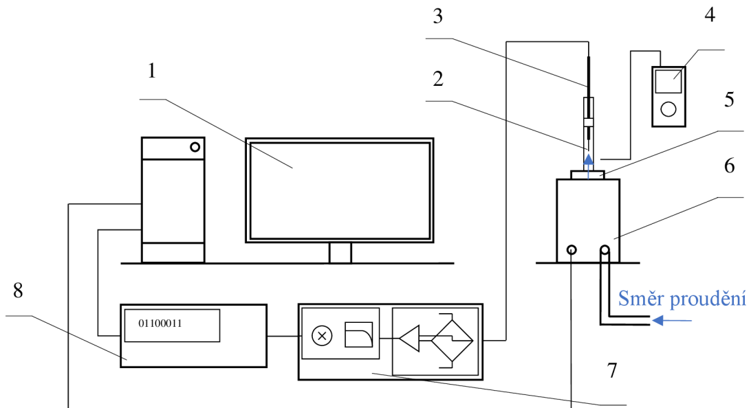
Obr. 3.1.2 Schéma experimentálního zařízení
