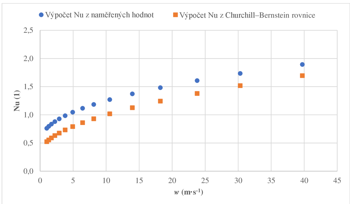
Obr. 4.2.3 Grafická závislost Nusseltova čísla na rychlosti proudění pro \alpha = 0,6
