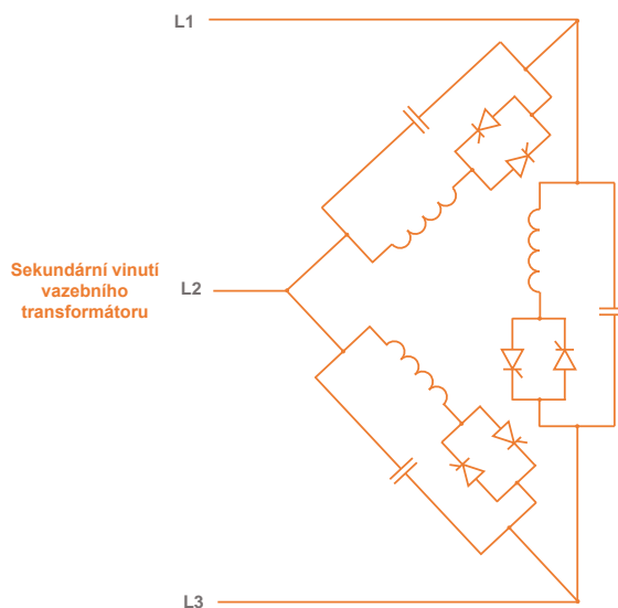
Obrázek 4 Schéma zapojení SVC, překresleno z [13].
