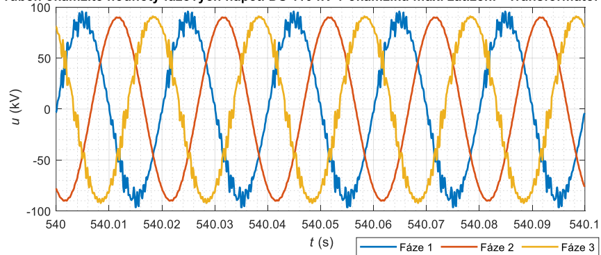
Průběh okamžité hodnoty fázových napětí DS 110 kV v okamžiku max. zatížení - Transformátor do "T"
