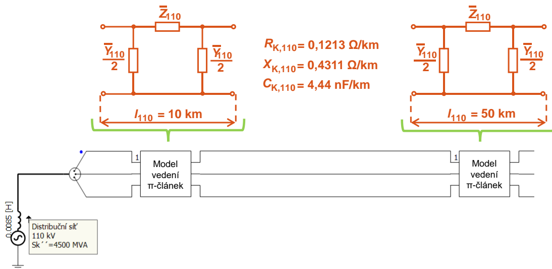
Obrázek 28 Model realistické testovací DS 110 kV.
