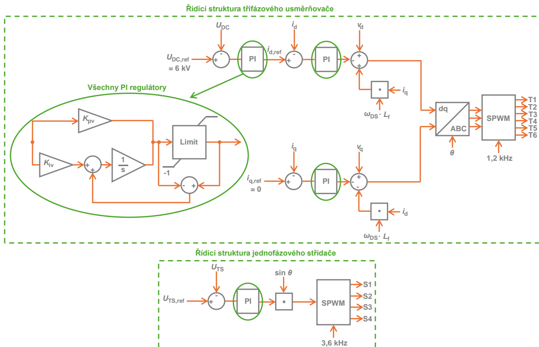
Obrázek 26 Řídící struktura SFC měniče.
