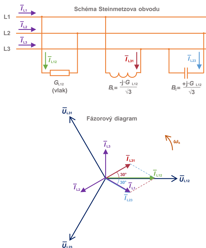
Obrázek 5 Princip Steinmetzova obvodu, překresleno z [14].
