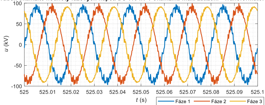
Průběh okamžité hodnoty fázových napětí DS 110 kV v okamžiku max. zatížení - Transformátor do "V"
