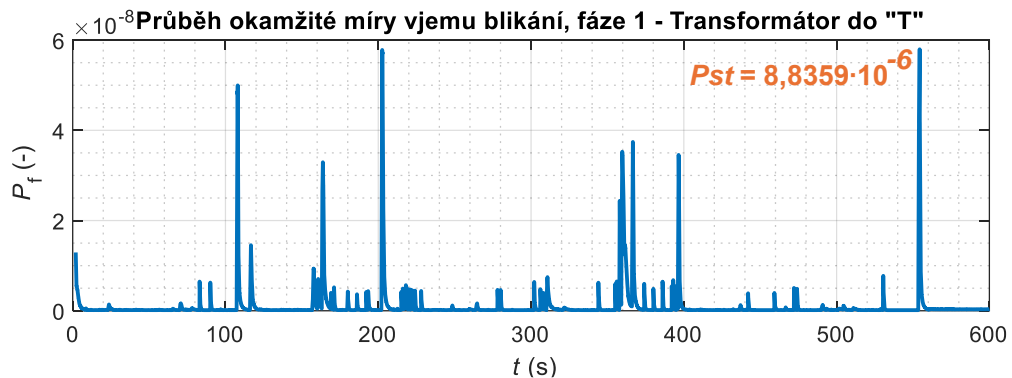
Obrázek 52 Průběh okamžité míry vjemu blikání – Transformátor do „T“.
