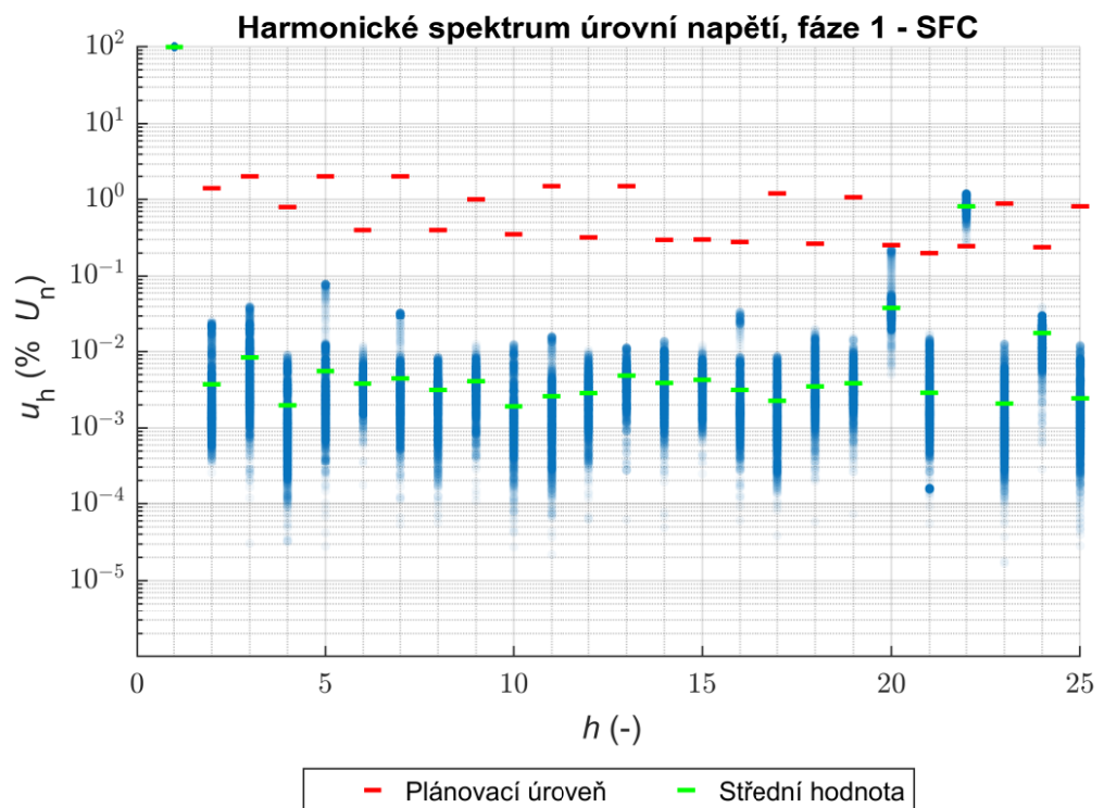
Obrázek 64 Harmonické spektrum úrovní napětí – SFC.
