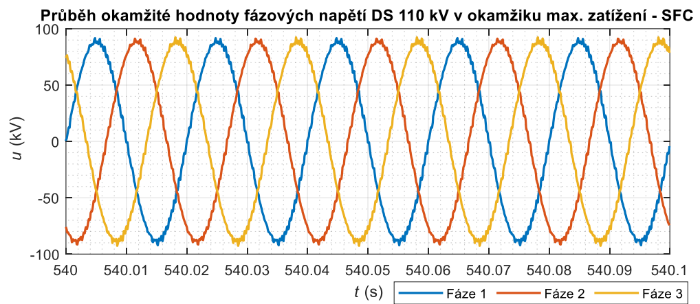
Obrázek 63 Průběh okamžité hodnoty fázových napětí DS při max. zatížení – SFC.
