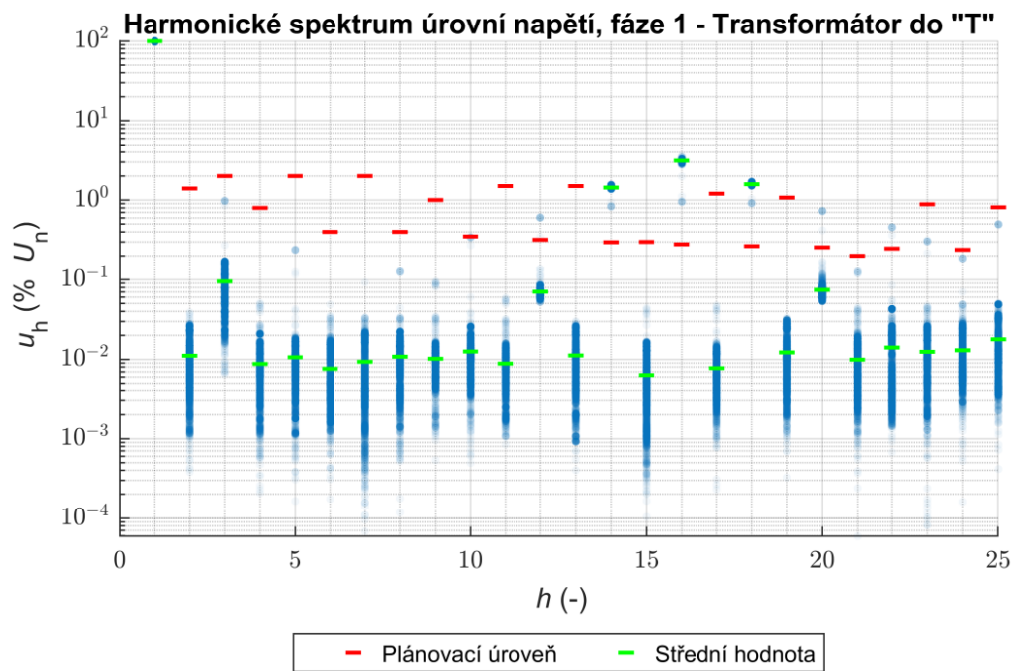
Obrázek 58 Harmonické spektrum úrovní napětí – Transformátor do „T“.
