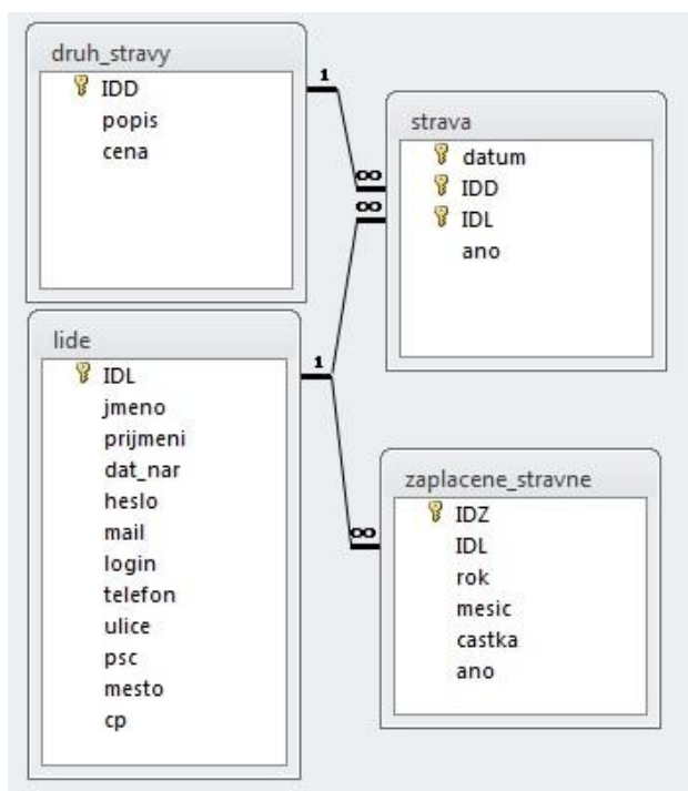
Obr. 5 - Schéma propojení tabulek 1
