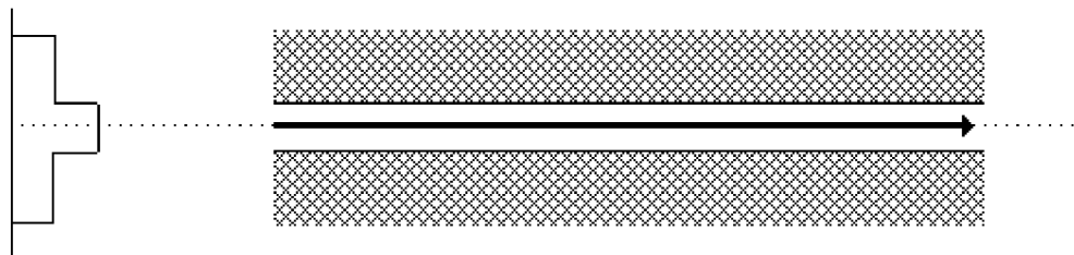
Obr. 14: Průběh indexu lomu step index u jednovidového vlákna. (9)
