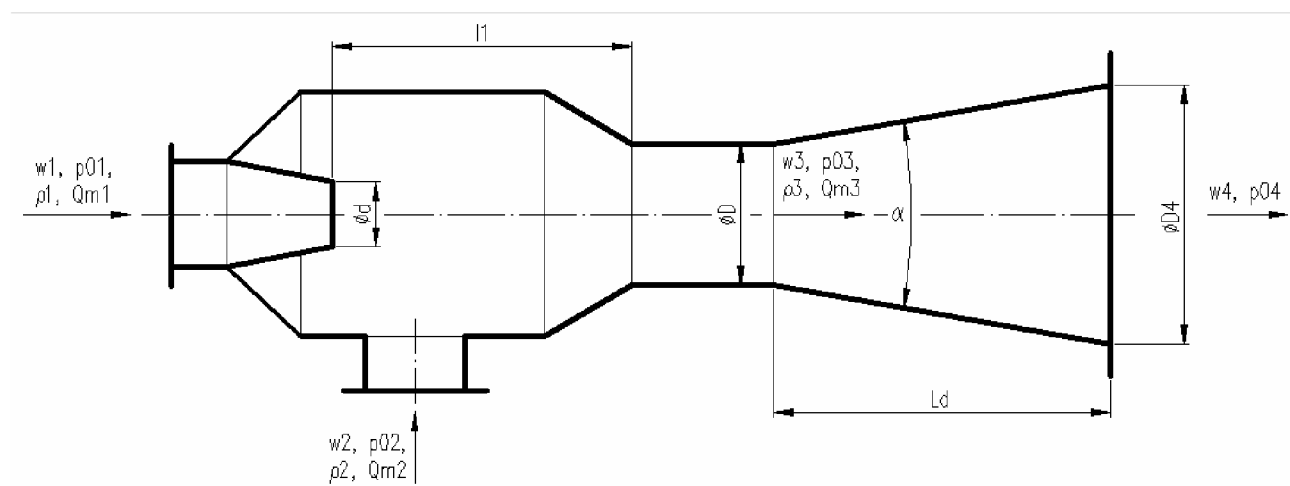
Obr. 22. Náčrtek ejektoru řešeného metodou CFD [18].
