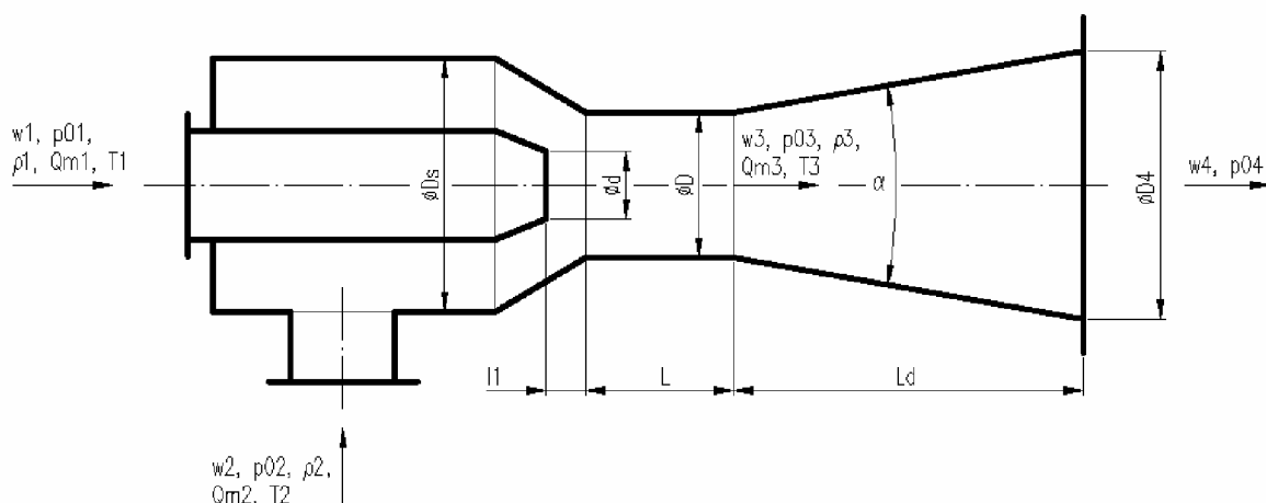
Obr. 20. Nákres ejektoru pro výpočet plynového ejektoru s podkritickým prouděním dle [1].
