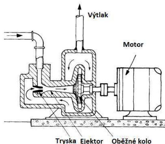
Obr. 8. Řez samonasávacím čerpadlem [8].
