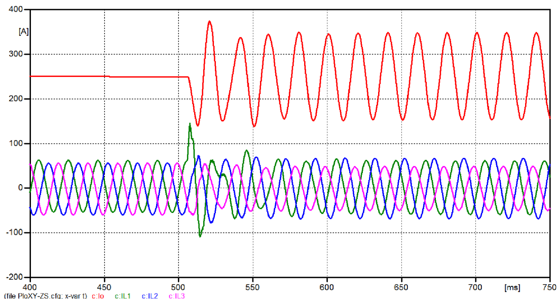
Obr. 6-6: Průběhy proudů při ZS (diplomová práce [22], 0 Ω)
