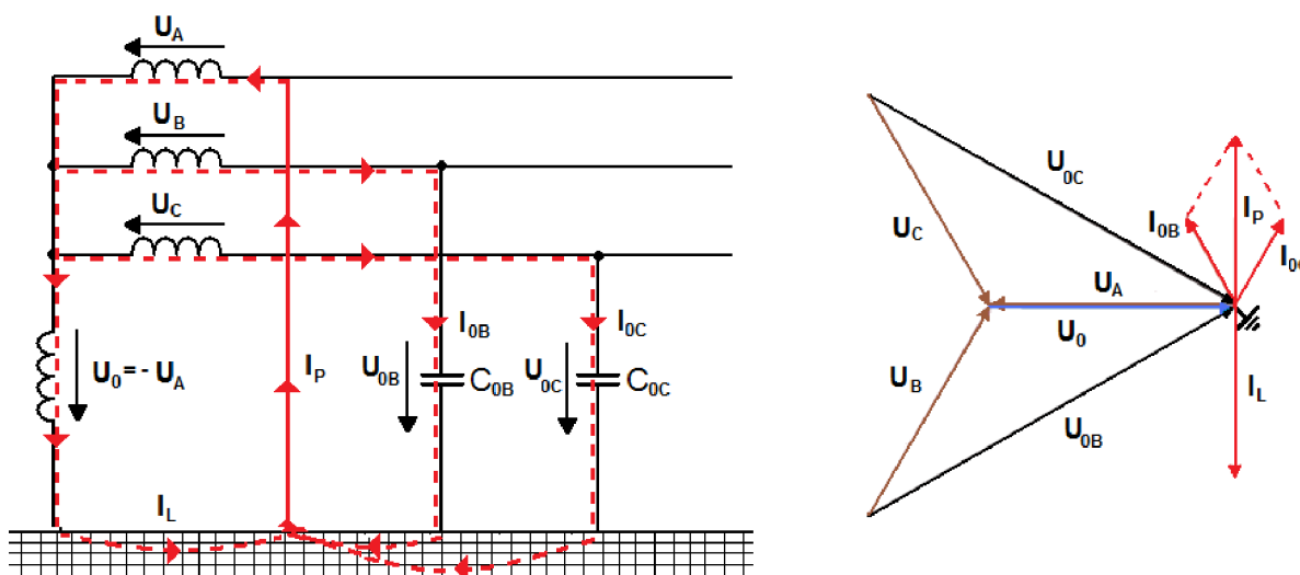
Obr. 2-1: Kompenzovaná síť [1]
