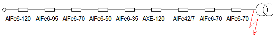
Obr. 6-2: Simulovaný vývod Kasejovice [22]
