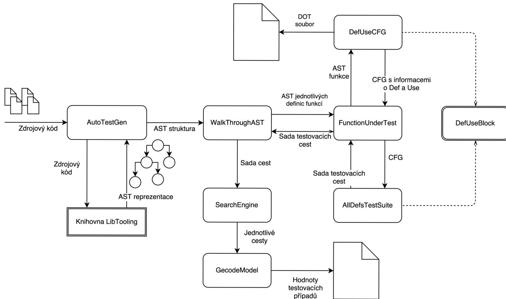
Obrázek 4.4: Vstupem aplikace je zdrojový kód (vlevo). Aplikace se napojí na Clang pomocí Visitoru, získá AST reprezentaci, kterou dále analyzuje třídami z knihovny LibTooling. Jednotlivé funkce jsou reprezentovány třídou FunctionUnderTest, u které je nejdříve vytvořen CFG, poté aplikováno kritérium pokrytí. Sada cest této funkce jde do GecodeModel modulu, ze kterého získáme hodnoty pro jednotlivé testovací případy, ze kterých jsou následně vytvořeny testovací případy.
