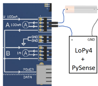
Obrázek 4.7: Zapojení
