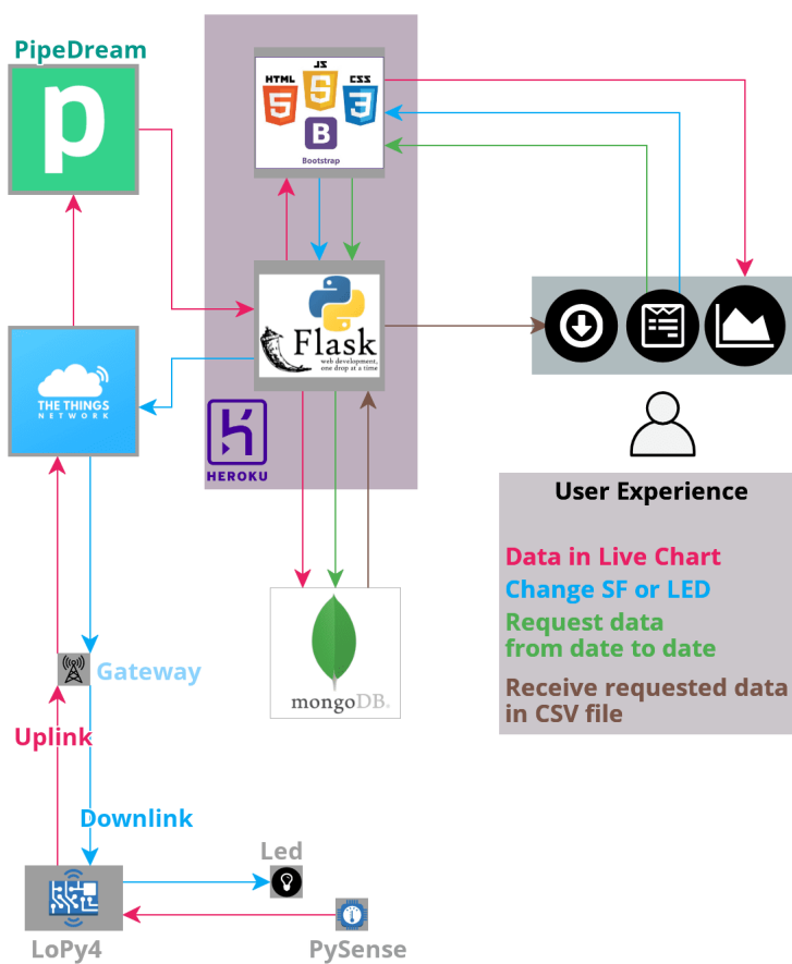
Obrázek 3.1: Architektura projektu
