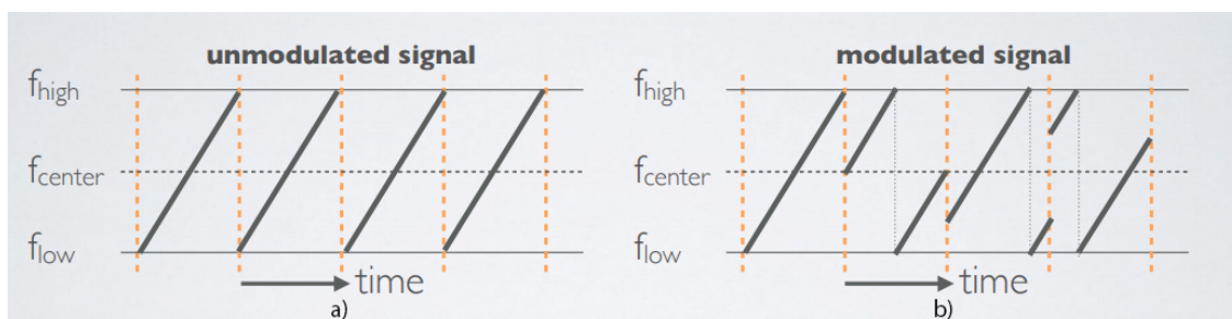
Obrázek 2.3: Modulace LoRa signálu a) nedomulovaný signál b) modulovaný signál
