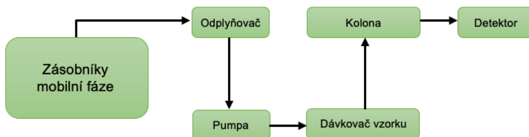
Obrázek 3: uspořádání jednotlivých komponent v HPLC systému
