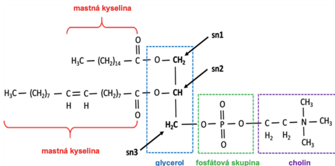
Obrázek 1: struktura fosfatidylcholinu, označení sn 1, 2, 3 znázorňuje pozice jednotlivých substituentů, převzato a upraveno dle MacDonald et al. 2019
