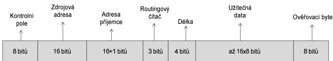
Obrázek 9: Struktura telegramu TP1 [2]
