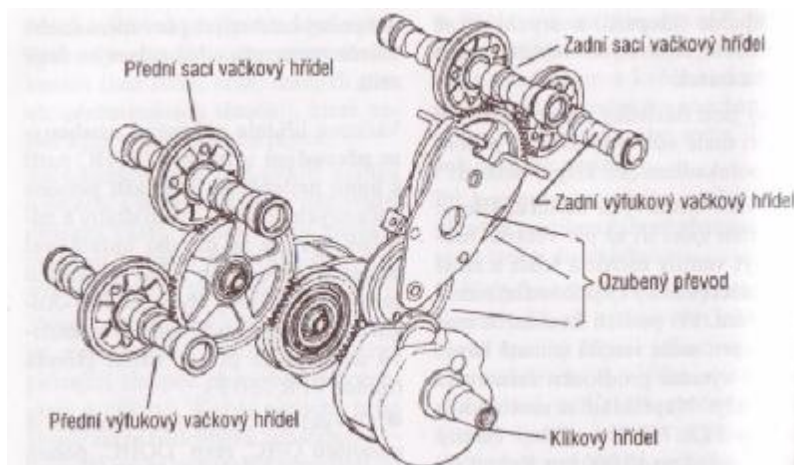
Obr. 3-12 Ventilový rozvod DOHC s ozubeným převodem (Honda VFR)
