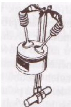
Obr. 3-13 Schéma rozvodu OHV
