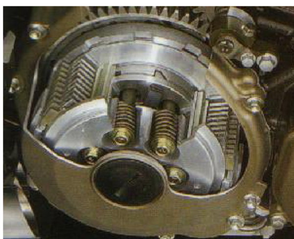
Obr. 3-16 Mokrá vícnelamelová spojka (Kawasaki Ninja 636)
