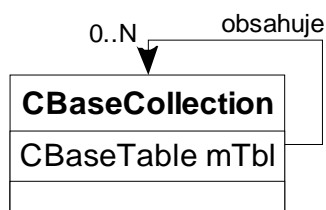
Obrázek 17: Rekurzivní definice bazové kolekce.
