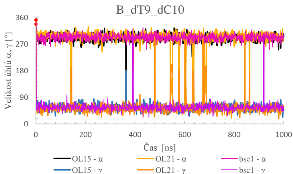
Obrázek 25: Graf úhlů \alpha a \gamma konformeru BB15 (rezidua: dT9_dC10) pro strukturu Ets domény vázající TGF- \beta receptor (3JTG). Východí krystalové hodnoty se v simulaci neudržely a byly nahrazeny hodnotami \alpha \sim 300^\circ a \gamma \sim 80^\circ (BB00).
