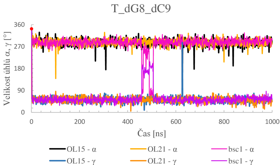
Obrázek 29: Graf úhlů \alpha a \gamma konformeru BB15 (rezidua: dG8_dC9) pro strukturu \lambda cII-aktivátor transkripce (1ZS4).
