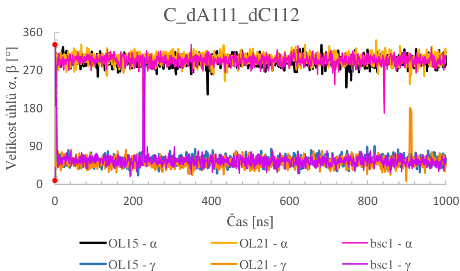
Obrázek 28: Graf úhlů \alpha a \gamma konformeru BB15 (rezidua: dC114_dC115) pro strukturu Ets domény vázající TGF- \beta receptor (3JTG). Poslední graf patřící struktuře 3JTG potvrzuje stejně jako grafy předešlé, že se hodnoty odpovídající konformeru BB15 neudržely.
