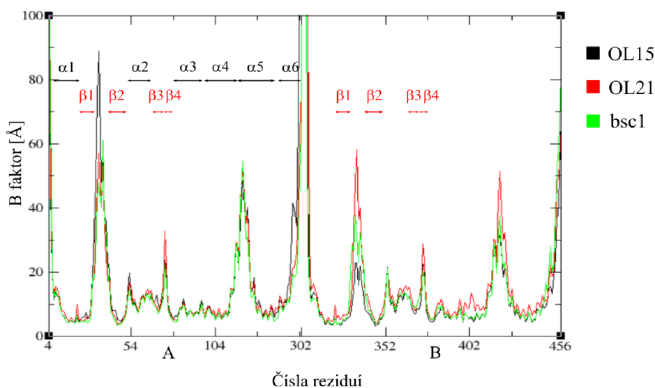
Obrázek 23: Graf B faktoru komplexu TATA boxu (IT9I) pro všechna silová pole.
