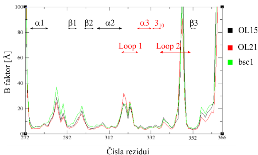
Obrázek 14: B faktor komplexu E1f3 s TGF- \beta receptorem (3JTG) pro všechna silová pole.
