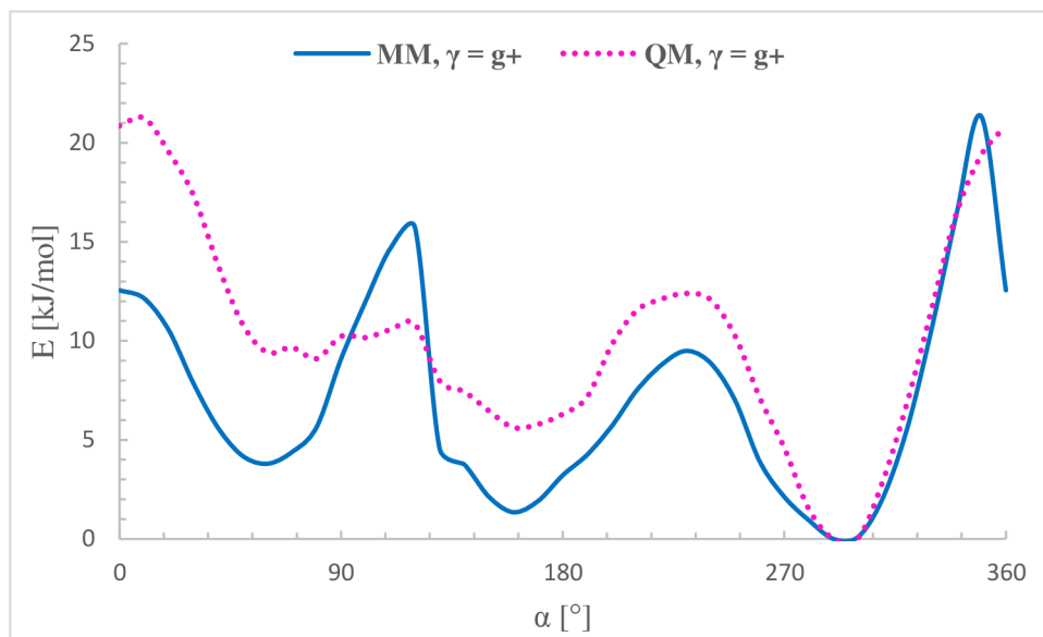
Obrázek 35: Torzní potenciály MM a QM pro torzi \alpha ( s \gamma nastavenou na g+ ). Energetická minima v hodnotách okolo 60^\circ , 170^\circ a 280^\circ .
