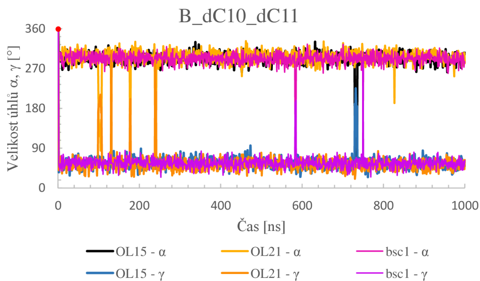
Obrázek 26: Graf úhlů \alpha a \gamma konformeru BB15 (rezidua: dT10_dT11) pro strukturu Ets domény vázající TGF- \beta receptor (3JTG). Východí krystalové hodnoty se v simulaci neudržely a byly nahrazeny hodnotami \alpha \sim 300^\circ a \gamma \sim 70^\circ (BB00).
