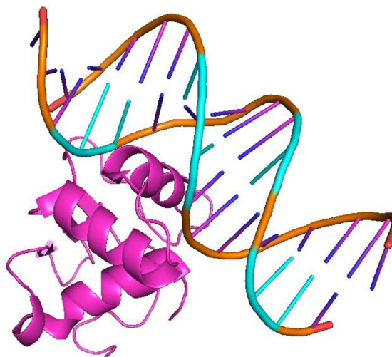
Obrázek 6: Struktura 3JTG vytvořena v programu PyMOL. Růžová barva znázorňuje protein a tyrkysová konformery BB15.
