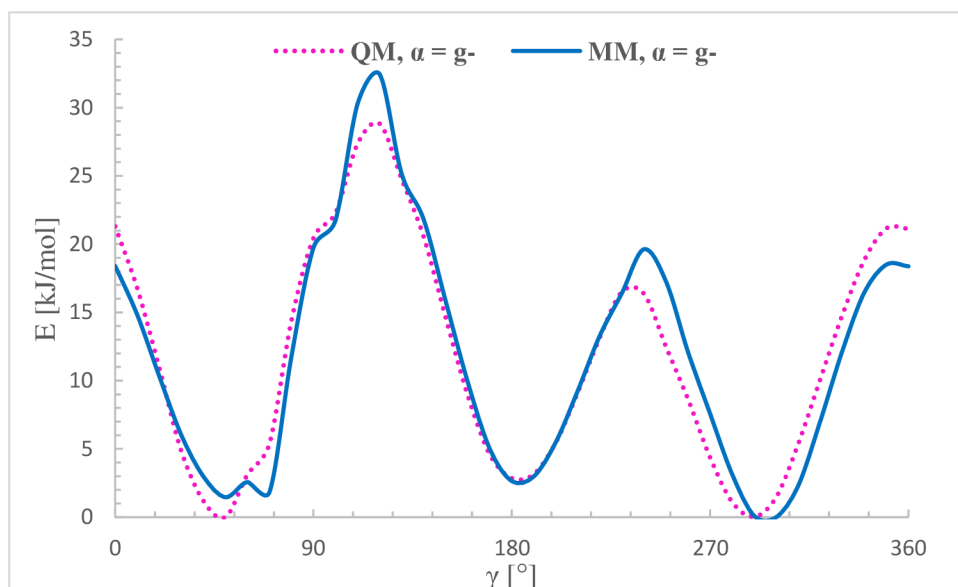
Obrázek 36: Torzní potenciály MM a QM pro torzi \gamma ( s \alpha nastavenou na g- ). Energetická minima v hodnotách okolo 60^\circ , 180^\circ a 280^\circ .
