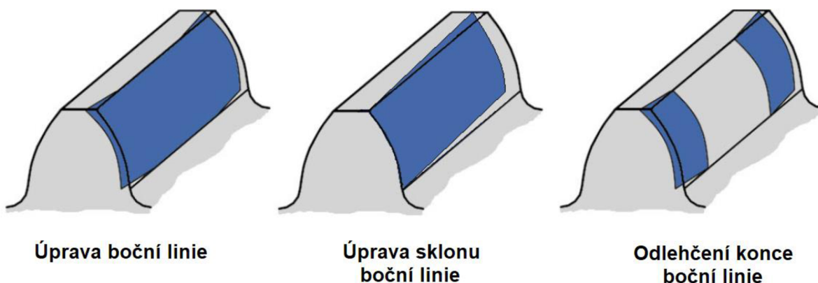
Obr. 28: Porovnání typů úprav bočních linií [12]
