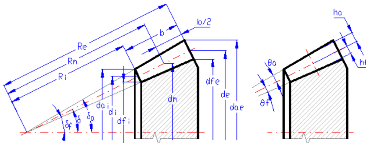
Obr. 16: Základní rozměry kuželového soukolí [6]
