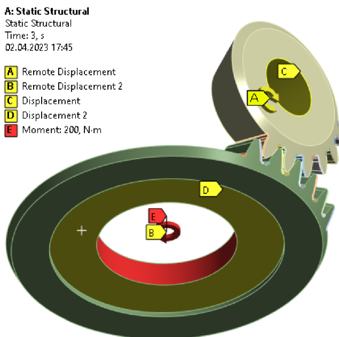
Obr. 40: Aplikace okrajových podmínek
