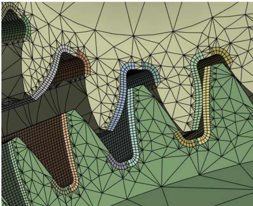
Obr. 39: Zjemnění síť v oblasti boků zubů
