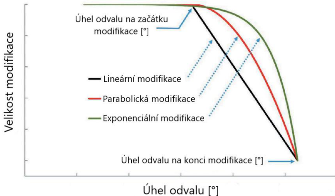
Obr. 26: Tvary výškové modifikace hlavy zuby [10]
