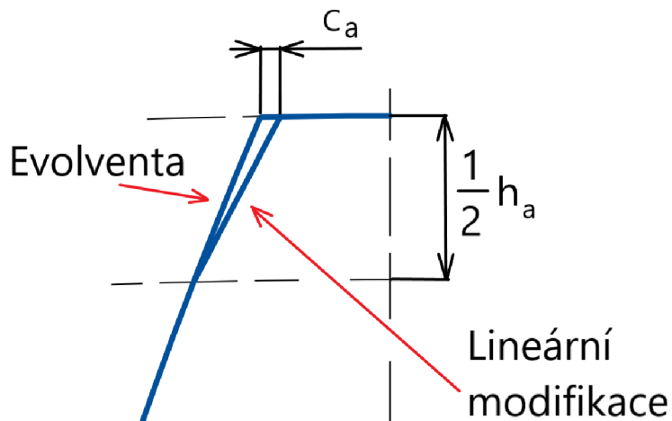
Obr. 41: Rozměry lineární modifikace
