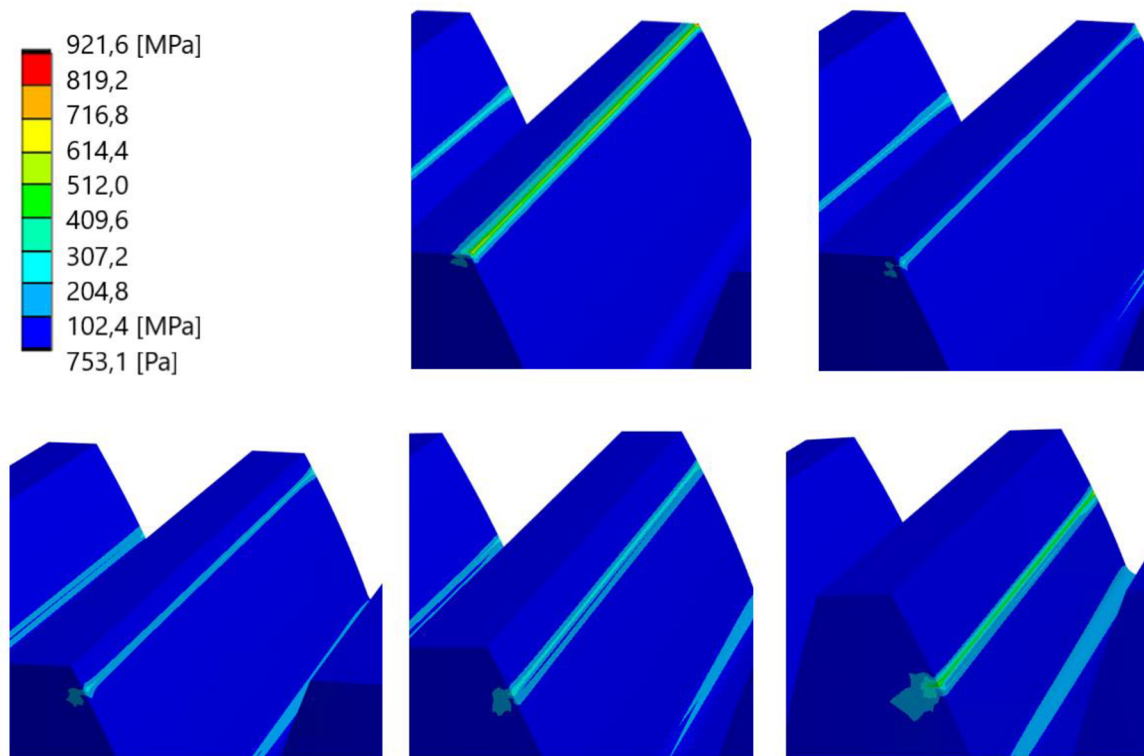
Obr. 32: Vstup sledovaného páru zubů do záběru
