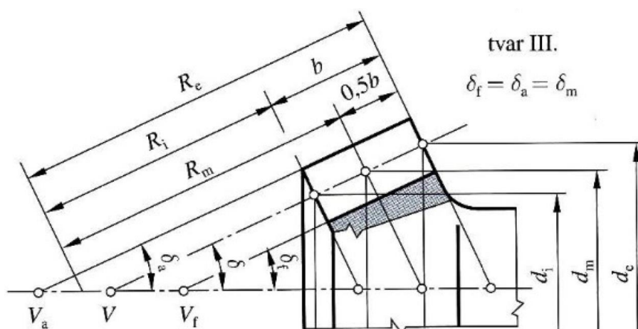
Obr. 4: Tvar věnce III [2]
