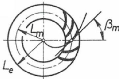
Obr. 15: Kuželové kolo se spirálovými zuby [3]
