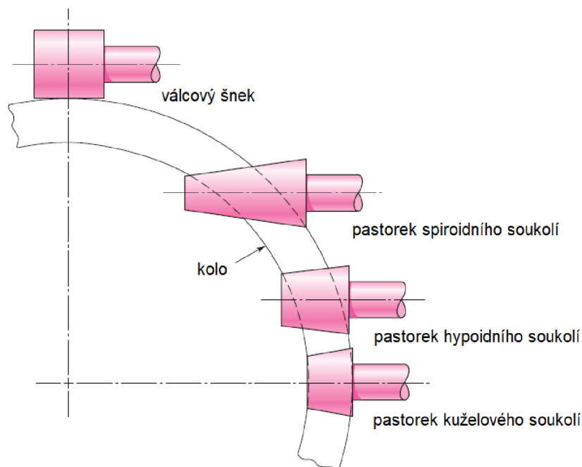
Obr. 1: Porovnání soukolí podle osy polohy pastorku [1]
