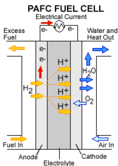
Obr. 7.7 - Schéma funkce PAFC [32]
