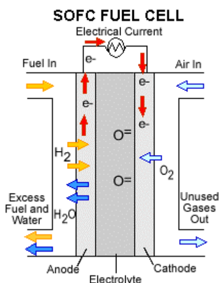
Obr. 7.9 - Schéma funkce SOFC [32]
