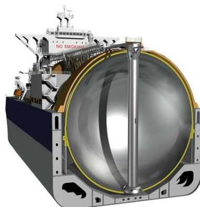
Obr. 5.1 - Řez tankerem pro převoz LNG [31]
