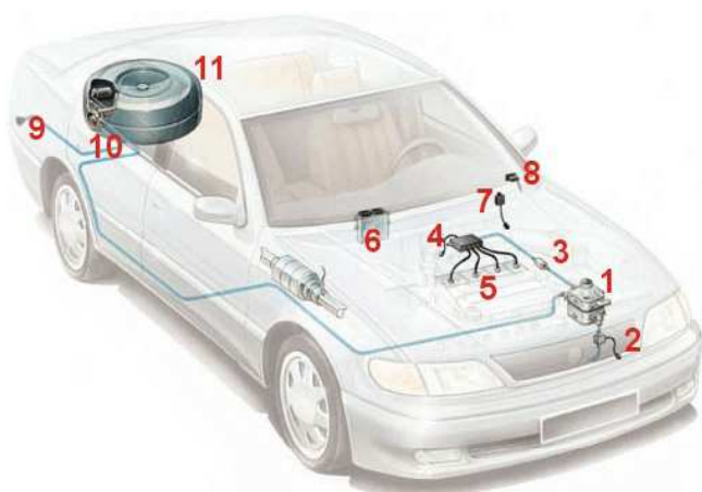
Obr. 4.4 - Zástavba s el. řízeným vícebodovým sekvenčním vstřikováním plynného LPG [2]
