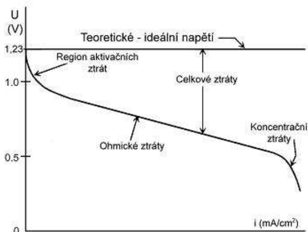
Obr. 7.4 - Ztráty v reálném palivovém článku [34]
