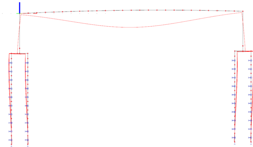
Obrázek 19 - Deformovaná konstrukce – model s pružným podepřením
