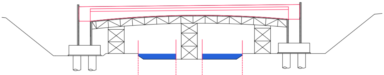
Obrázek 50 - Fáze 3 - Zapažení vodního toku, výstavba skruže a následná betonáž mostovky
