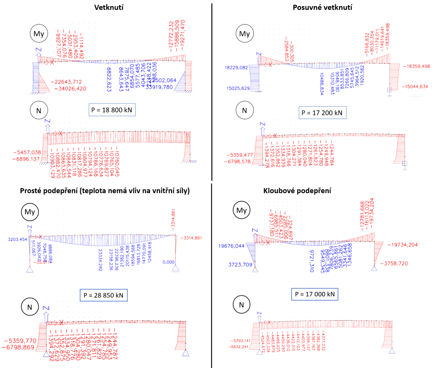
Obrázek 17 - Srovnání rovinných modelů
