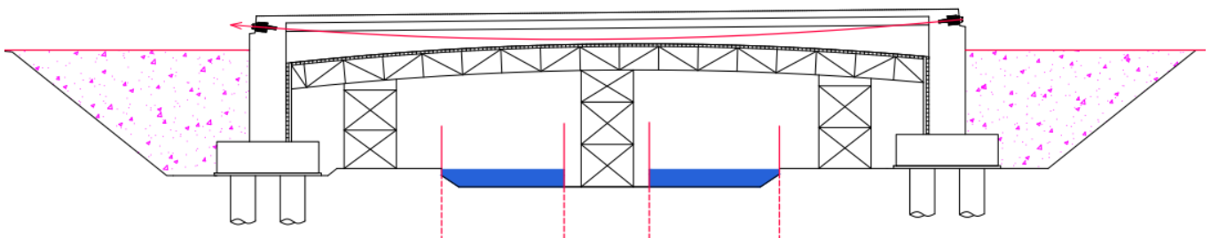
Obrázek 51 - Fáze 4 - Zасыпání rubu opěr, napínání kabelů čas t_0
