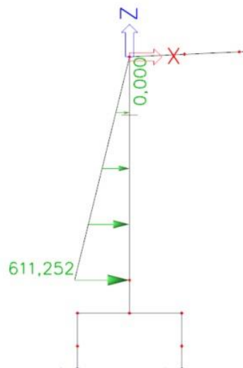
Obrázek 33 - Zemní tlak v čase t_\infty (stojka č.1)
