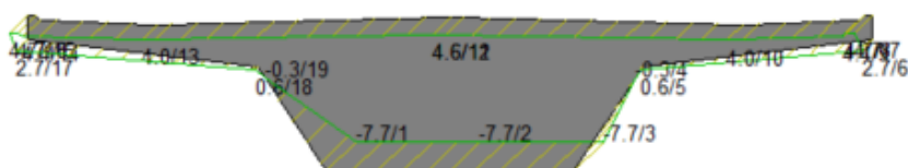
Obrázek 26 - Napětí v rámovém rohu (nad podporou)
