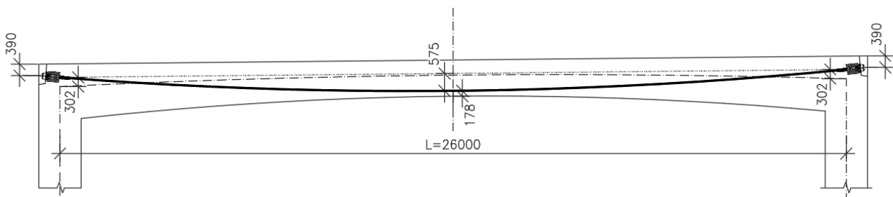
Obrázek 24 - Excentricity a vzepětí předpínacích kabelů
