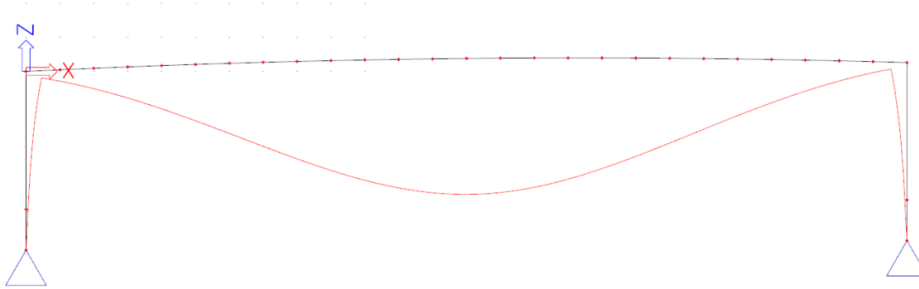
Obrázek 21 - Deformovaná konstrukce – kloubové podepření
