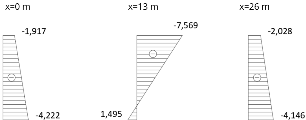
Obrázek 41 - Napětí v čase t^\infty - častá kombinace
