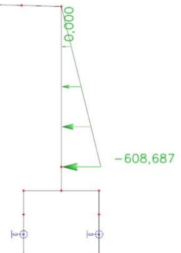
Obrázek 32 - Zemní tlak v čase t_\infty (stojka č.2)
