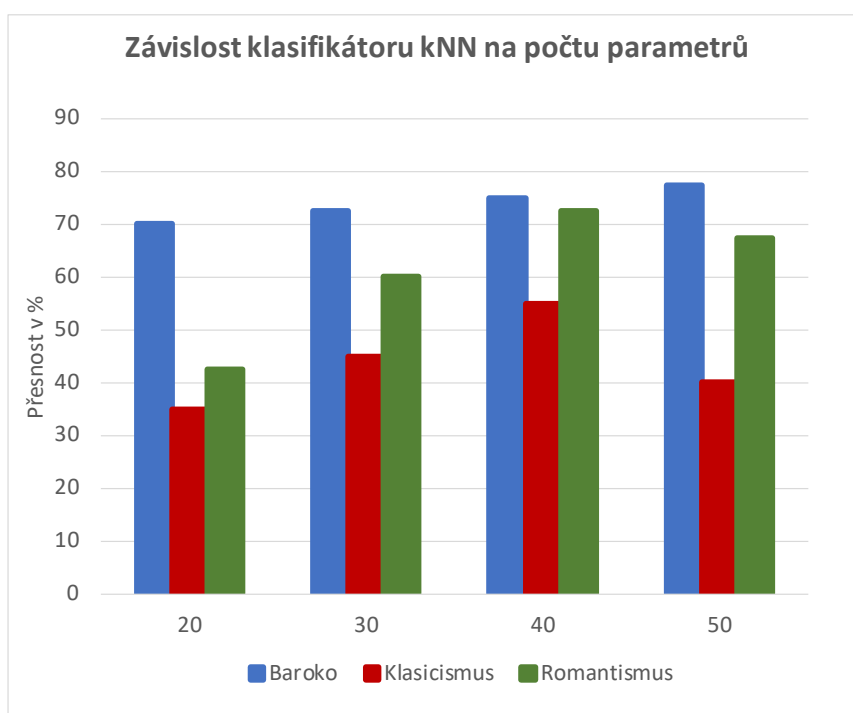
Obr. 6.4: Závislost přesnosti klasifikátoru kNN na počtu parametrů
