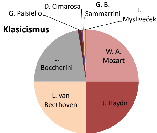
Obr. 2.6: Dataset: klasicismus
