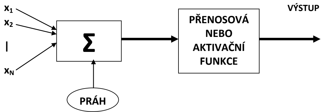
Obr. 3.4: Schéma neuronu
