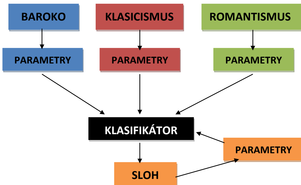
Obr. 3.1: Metoda MIR
