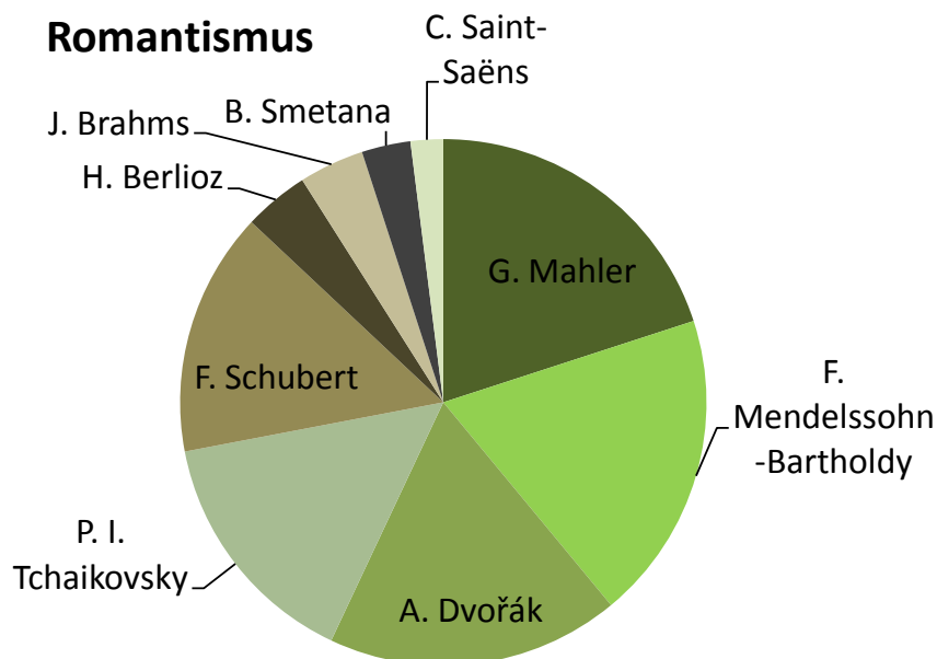
Obr. 2.7: Dataset: romantismus
