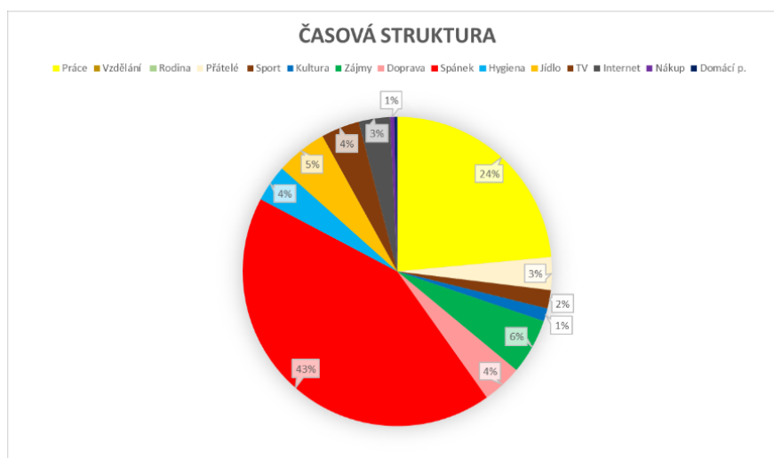
Graf 4 - procentuální vyjádření časových skupin v grafu (respondent 4)
