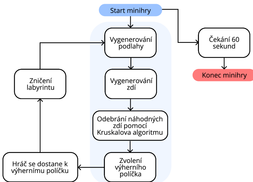
Obrázek 4.24: Nejdříve se vygenerují všechny buňky se všemi čtyřmi stěnami. Poté se odstraní náhodné stěny pomocí Kruskalova algoritmu. Posledně se odstraní jedno políčko podlahy, do kterého se hráč musí dokutálet pro vygenerování nového labyrintu.
