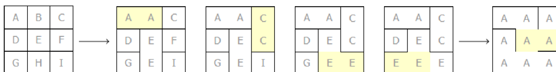
Obrázek 4.25: Ukázka, jak funguje Kruskalův algoritmus při generování labyrintu. Jednotlivé buňky jsou svůj vlastní podstromeček. Každá buňka se odstraní náhodná zeď za podmínky, že buňka, s kterou sdílí danou stěnu není ze stejného podstromečku. Obrázek převzatý 4 .
