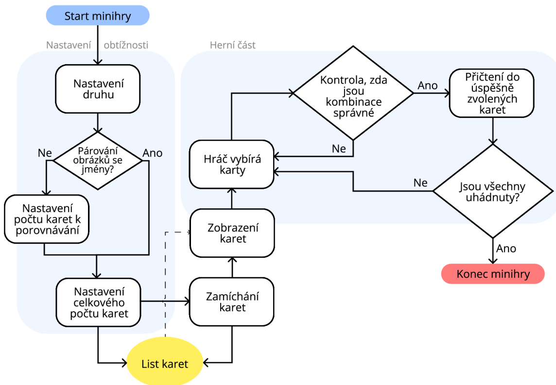
Obrázek 4.19: Po spuštění minihry si nejdříve hráč nastaví druh pexesa. Pokud si zvolil spojování obrázků s obrázky, může si navíc nastavit kolik stejných karet chce spojovat, páry nebo trojice. Konečným nastavením je celkový počet druhů. Po dokončení nastavení se karty zamíchají a vloží do listu karet. Hráč nyní otáčí karty. Pokud se snaží spojovat dvojice, kontroluje se vždy po otočení druhé karty. Pokud se spojují trojice, karty se kontrolují po otočení druhé a třetí karty. Pokud se najde správná kombinace, zkontroluje se, zda byly všechny karty otočeny. Aby hráč nemusel při opakovaném hraní vždy měnit nastavení, je umožněno si nastavení zachovat i pro příští hru.
