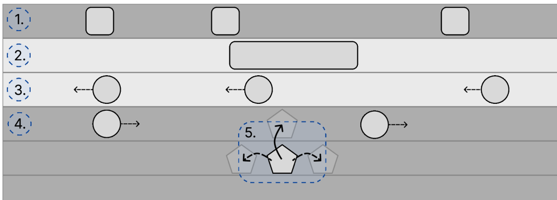
Obrázek 4.15: Jeden označený řádek reprezentuje jedno herní pole. Objekty statického zemního pole vyznačené na obrázku číslem jedna jsou kameny, které brání žabákovi v pohybu. Žabák přes ně nemůže skákat jak ze předu, tak ani z boku. Na jednom poli se vždy vyskytují tři kameny. Obdobně na vodním statickém poli, vyznačeným číslem dva, se vyskytují objekty v podobě stromového kmene. Ten bývá v poli jediný. Pozice objektů u statických polí jsou náhodné. Pole číslo tři reprezentuje vodní pole s hýbající se mi objekty – lekníny. Posledním druhem pole je zemní pole s pohybující se mi hlemýždí. Směr pohybu po sobě jdoucích polí je vždy opačný. Na obrázku jsou číslem pět také vyznačeny pohyby, které hráč může vykonat.
