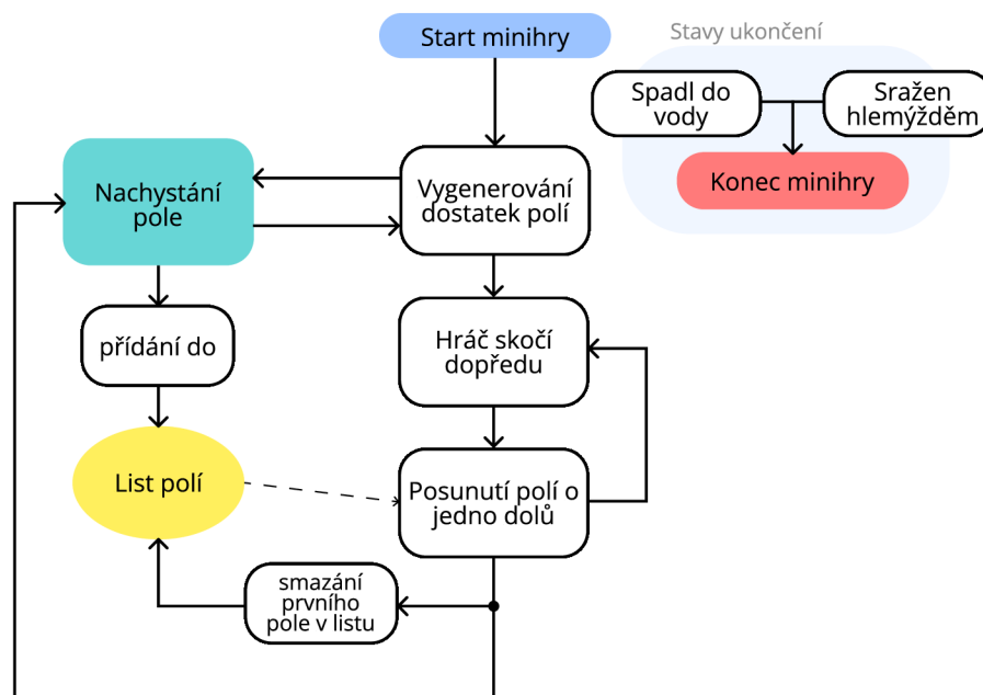
Obrázek 4.16: Na začátku minihry se musí vygenerovat dostatek polí na zaplnění celé obrazovky. Pokaždé, jak se hráč posune o pole dopředu, se smaže první pole v listu a zároveň se na konec listu přidá nové nachystané pole. Hra se ukončí pokud hráč spadne do vody nebo pokud ho srazí hlemýžděm.
