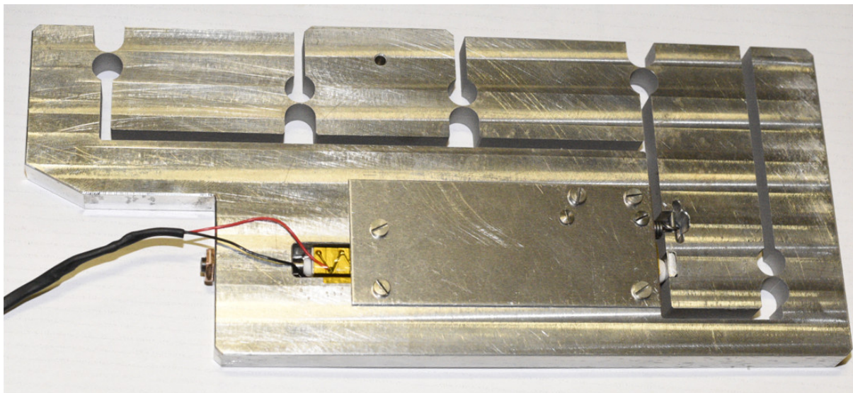
Obrázek 4.2: Sestava piezo aktuátoru pro pohyb v ose z .
