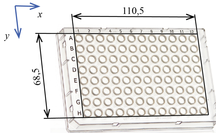
Obrázek 1.6: Efektivní rozměry mikrotitrační destičky. Převzato a upraveno z [25]
