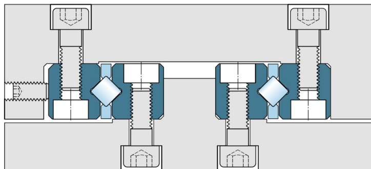
Obrázek 3.9: Vedení se zkříženými válečky. Dvojice vedení je proti sobě předeprnuta z levé strany stavěcími šrouby. Převzato z [32].
