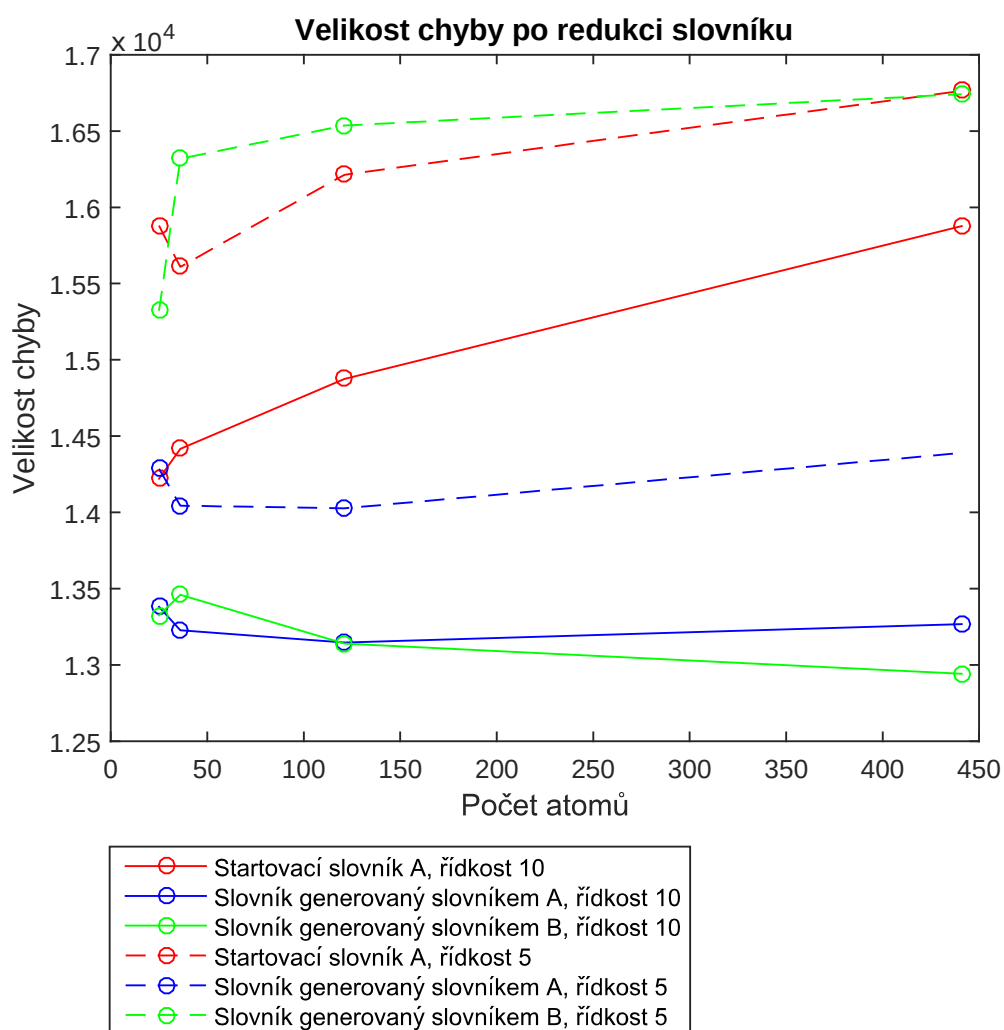
Obrázek 4.11: Porovnání velikostí chyby aproximace pro různé slovníky o různých velikostech – 25, 36, 121 nebo 441 atomů. Červená čára označuje fixní slovník, zelená a modrá natrénované.
