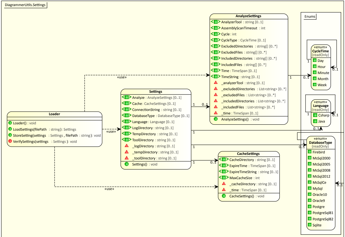
Obrázek A.3: Diagram tříd pro XML konfigurační soubor a práci s ním. Lze jej získat použitím parametrů dle http://ac-diagrammer.aspone.cz/DrawClass?source=DiagrammerUtils.Settings.**&image=svg&landscape=false
