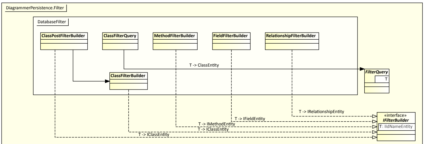
Obrázek A.4: Zjednodušený diagram tříd pro filtrování nad databází. Lze jej získat použitím parametrů dle http://ac-diagrammer.aspone.cz/DrawClass?source=DiagrammerPersistence.Filter.**&image=svg&style=normal&noParts=field,method&noRelationships=dependency
