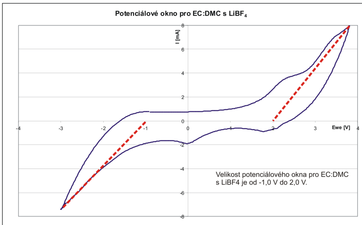
Obr. 54: Velikost potenciálového okna pro EC:DMC s LiBF 4
