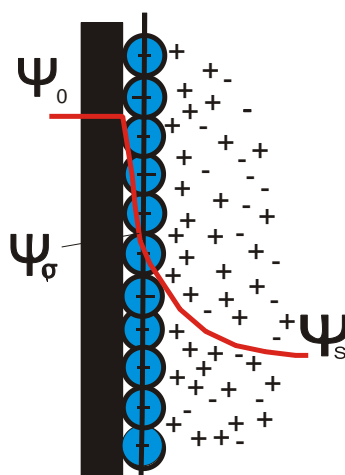
Obr. 7: Sternův model elektrické dvojrstvy, kde \psi_0 je velikost potenciálu na povrchu pevné fáze, \psi_s je hodnota potenciálu ve středu iontu na povrchu pevné fáze, \psi_\delta je velikost potenciálu ve vzdálenosti od povrchu pevné fáze[11]
