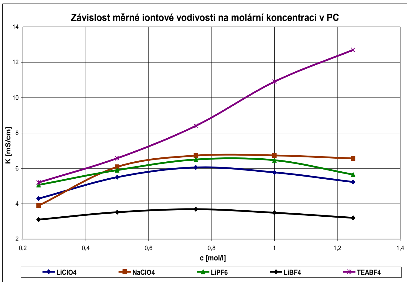
Obr. 23: Znávorňuje závislost měrné iontové vodivosti na molární koncentraci jednotlivých solí v propylenkarbonátu
