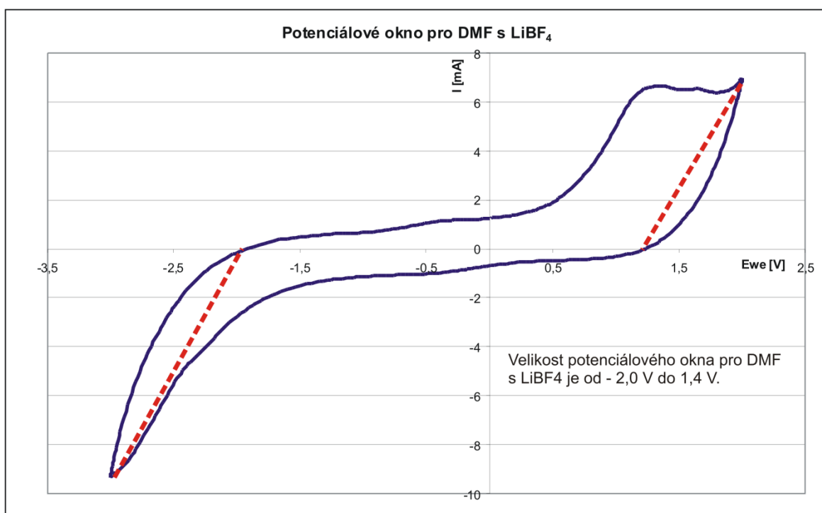
Obr. 39: Velikost potenciálového okna pro DMF s LiBF 4
