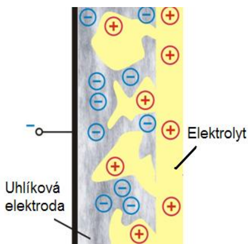
Obr. 4: Princip elektrické dvojvrstvy[14]
