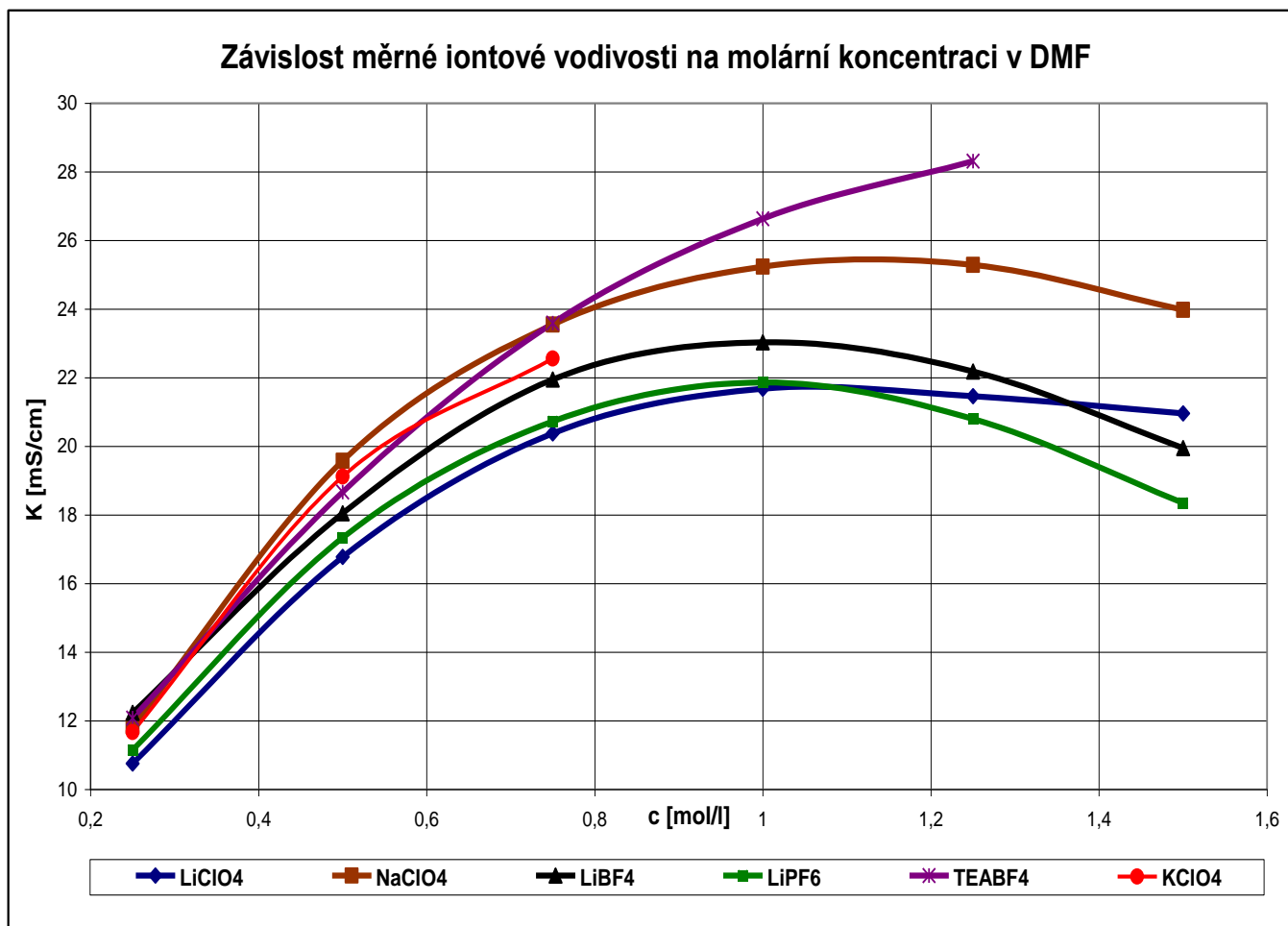
Obr. 24: Znávorňuje závislost měrné iontové vodivosti na molární koncentraci jednotlivých solí v N, N dimethylformamidu
