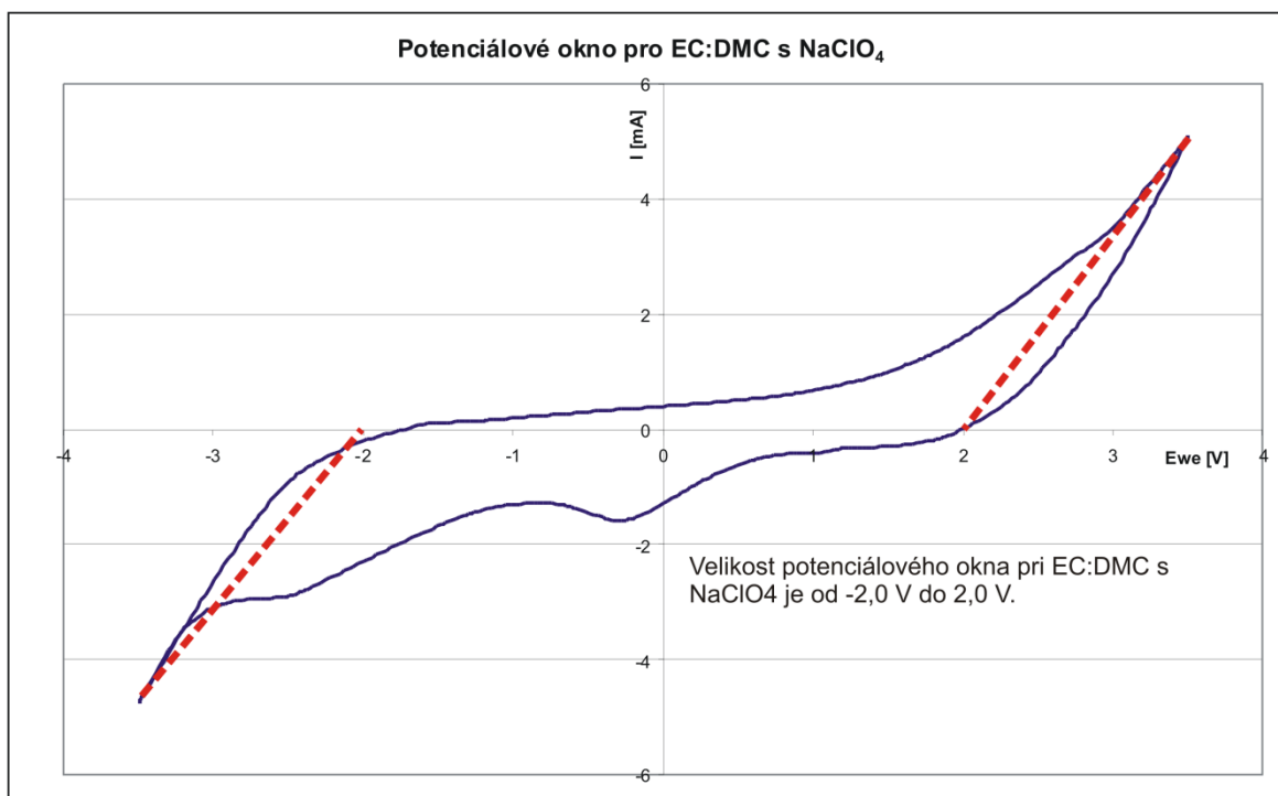
Obr. 53: Velikost potenciálového okna pro EC:DMC s NaClO 4
