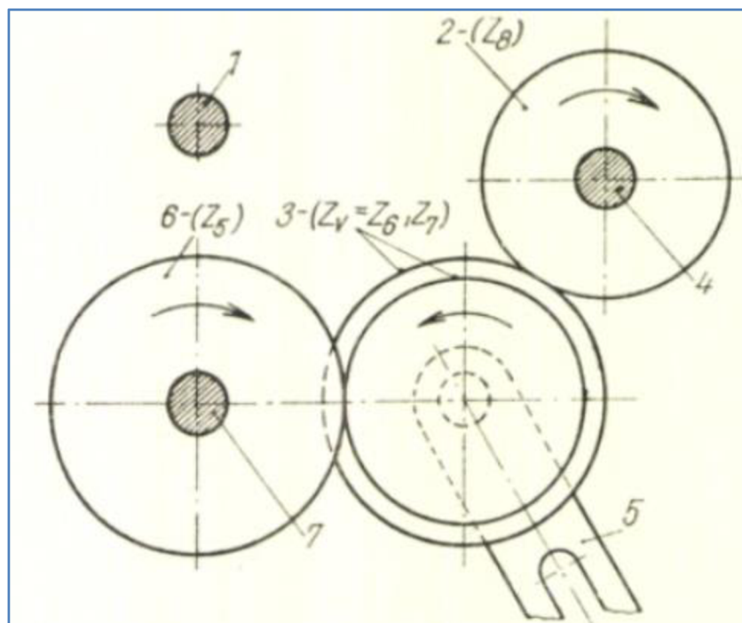
Obr. 2.17 Převodové soukolí s dvojitým převodem při tvorbě drážky s pravou šroubovicí. Legenda: 1 – vřeteno dělicího přístroje; 2 – hnané výměnné kolo Z_4 ; 3 – mezikolo Z_v ; 4 – hřídel kuželového kola; 5 – lyra kol; 6 – hnací výměnné kolo Z_5 ; 7 – posuvový šroub stolu frézky [5].
