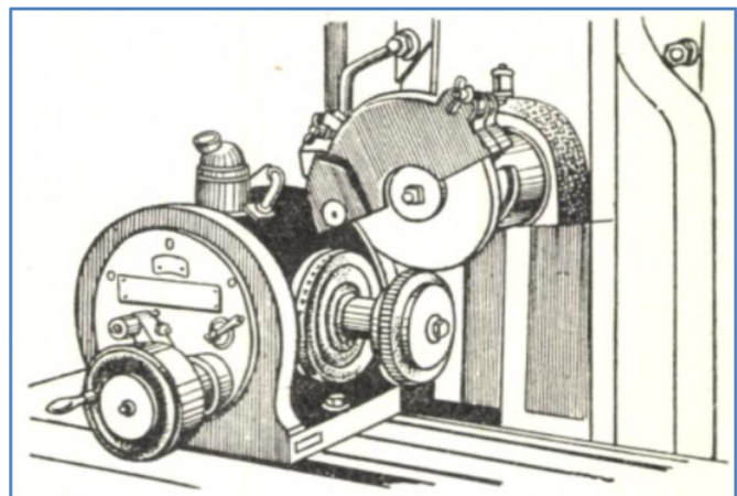
Obr. 2.26 Optický přístroj při broušení [5].
