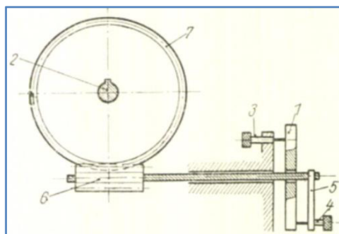
Obr. 2.8 Schéma seřízení dělicího pro sdrúžené dělení.
