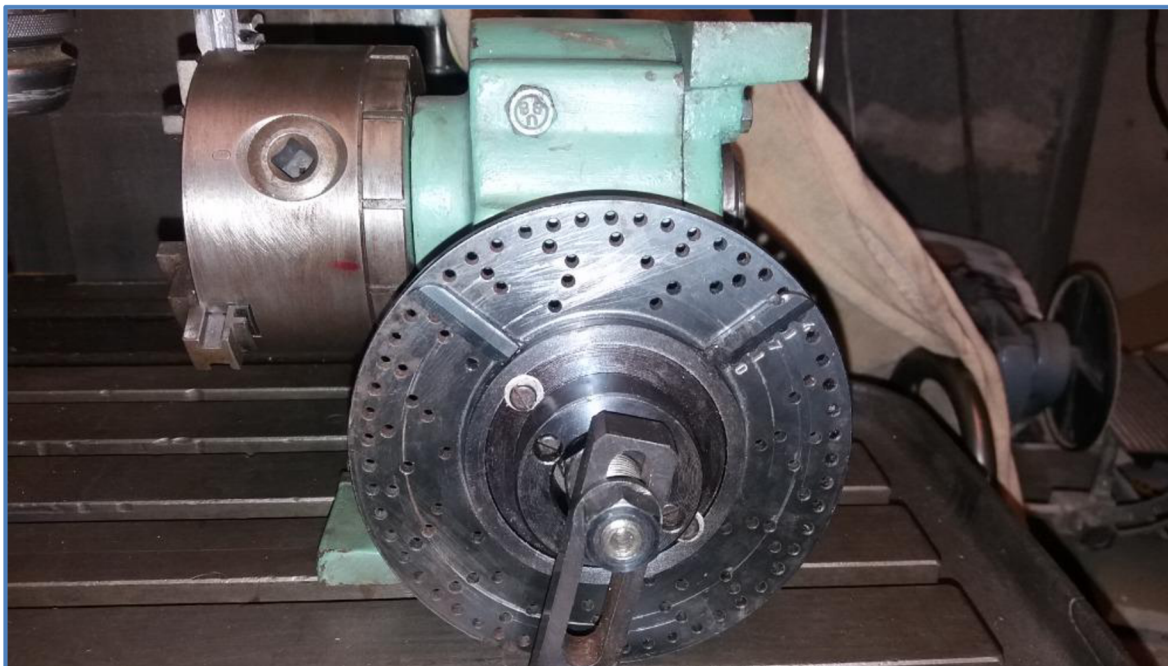
Obr. 1.0 Dělicí přístroj.
