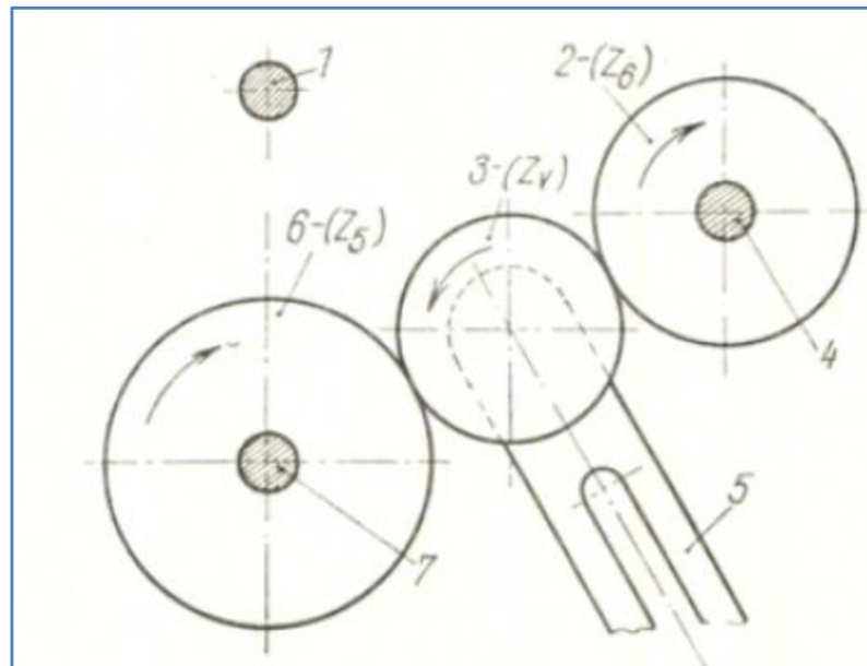
Obr. 2.16 Převodové soukolí s jednoduchým převodem při tvorbě drážky s pravou šroubovicí. Legenda: 1 – vřeteno dělicího přístroje; 2 – hnané výměnné kolo Z_4 ; 3 – mezikolo Z_v ; 4 – hřídel kuželového kola; 5 – lyra kol; 6 – hnací výměnné kolo Z_5 ; 7 – posuvový šroub stolu frézky [5].
