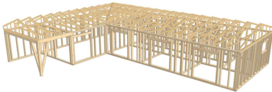
Obr. 17 Trojrozměrný model nosné konstrukce navrhovaného domu (vlastní zpracování)
