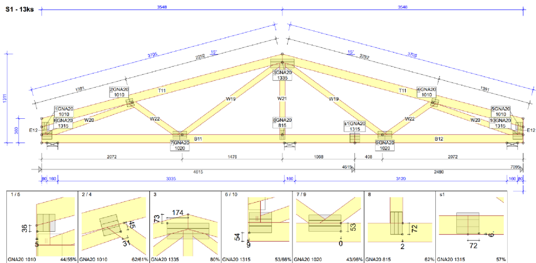
Obr. 20 Výrobní výkres vazníku S1 (vlastní zpracování)
