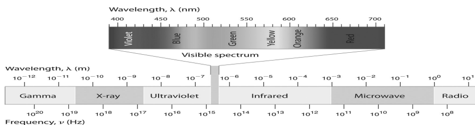
Obr. 10: Elektromagnetické spektrum [159].
