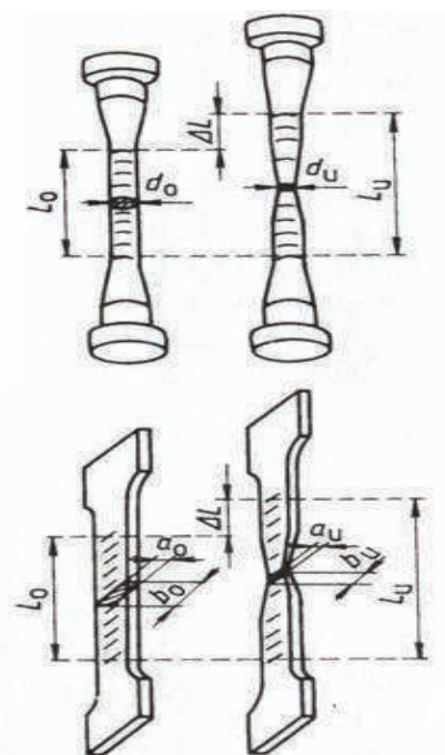
(1) Obr.4 Tvar vzorků [27]
