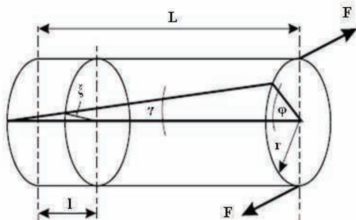
Obr.10 Schéma zkoušky krutem [19]
