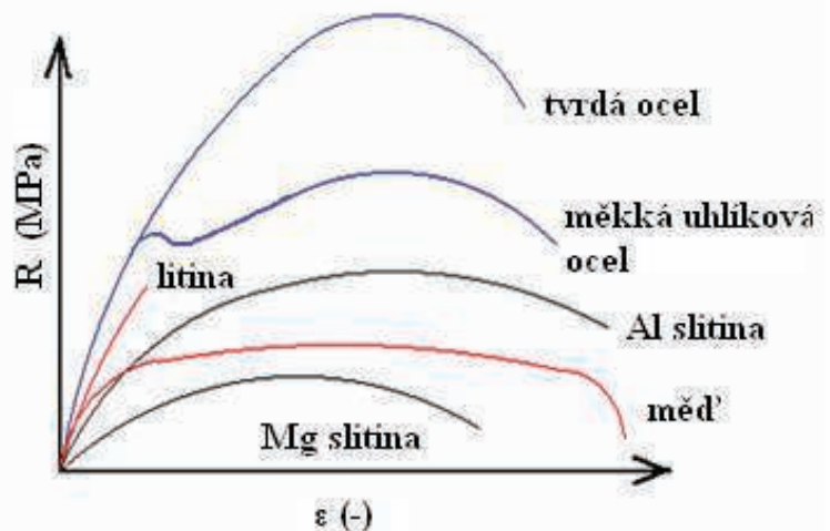
Obr. 6 Příklady diagramů pro různé materiály [8]
