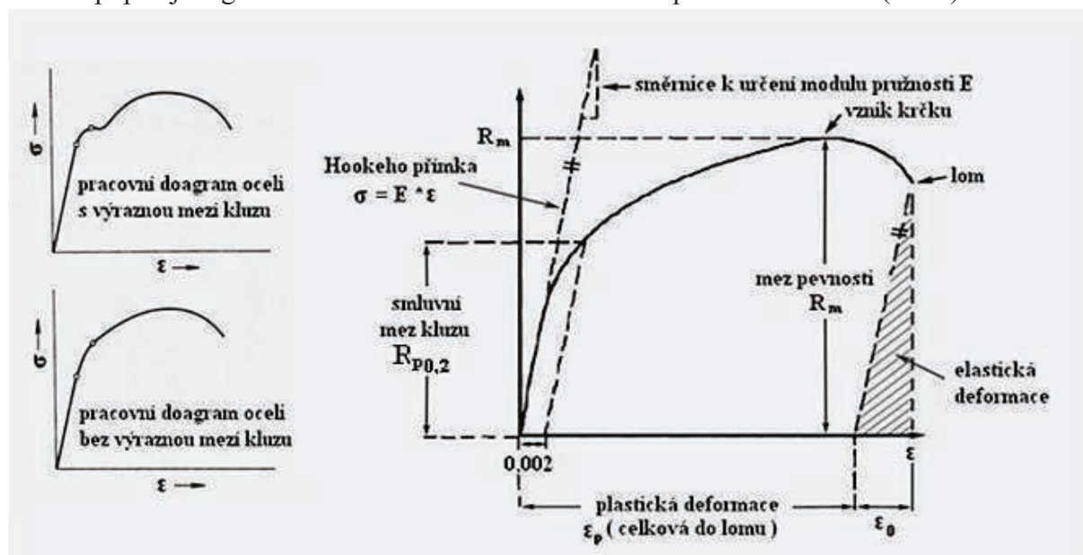
Obr. 5 Srovnání tahových diagramů s výraznou a nevýraznou mezí kluzu [ 27 ]
