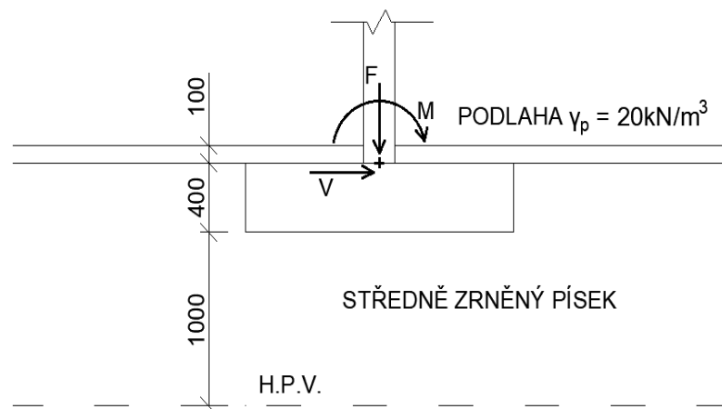
Obr. 6.1: Schéma zatížení
