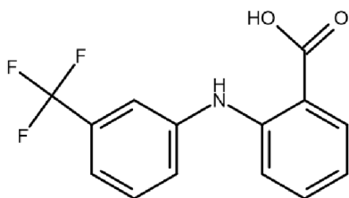
Obr. 4: Strukturální vzorec kyseliny niflumové (NIF)
