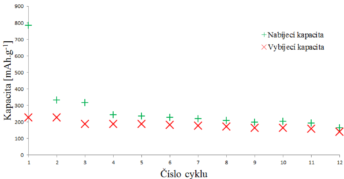
Obr. 58: Nabíjecí a vybíjecí kapacita každého cyklu přírodního grafitu COND 5995 lisovaného tlakem 100 \text{ kg.cm}^{-2}
