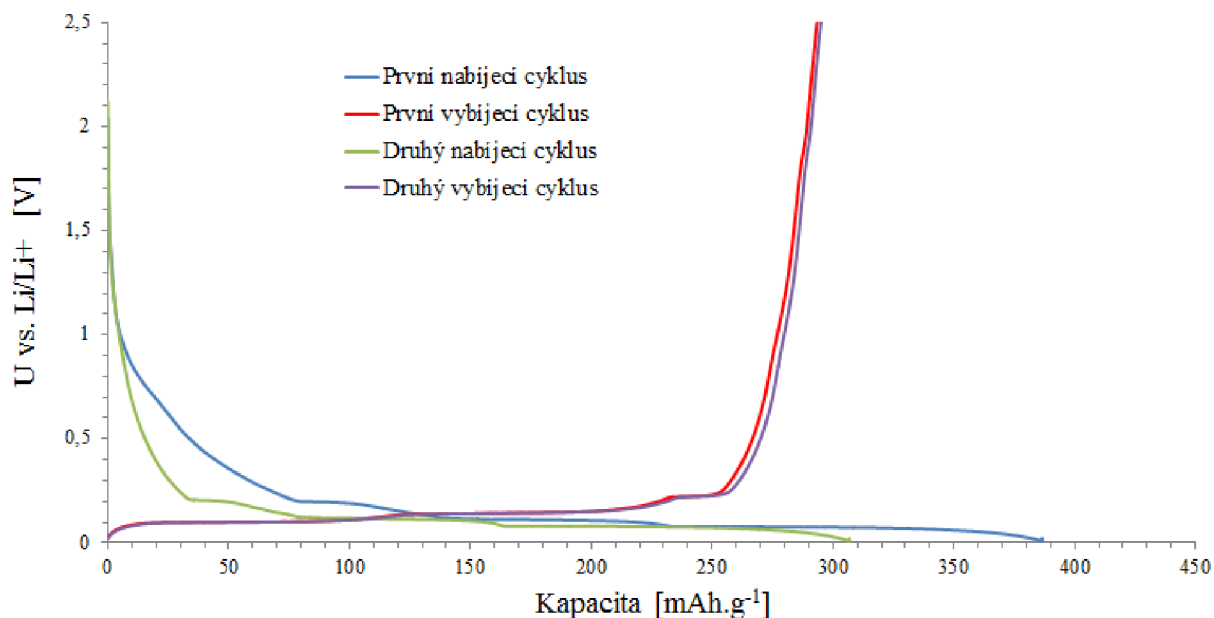
Obr. 33: První dva nabíjecí a vybíjecí cykly přírodního grafitu 280 H nelisovaného
