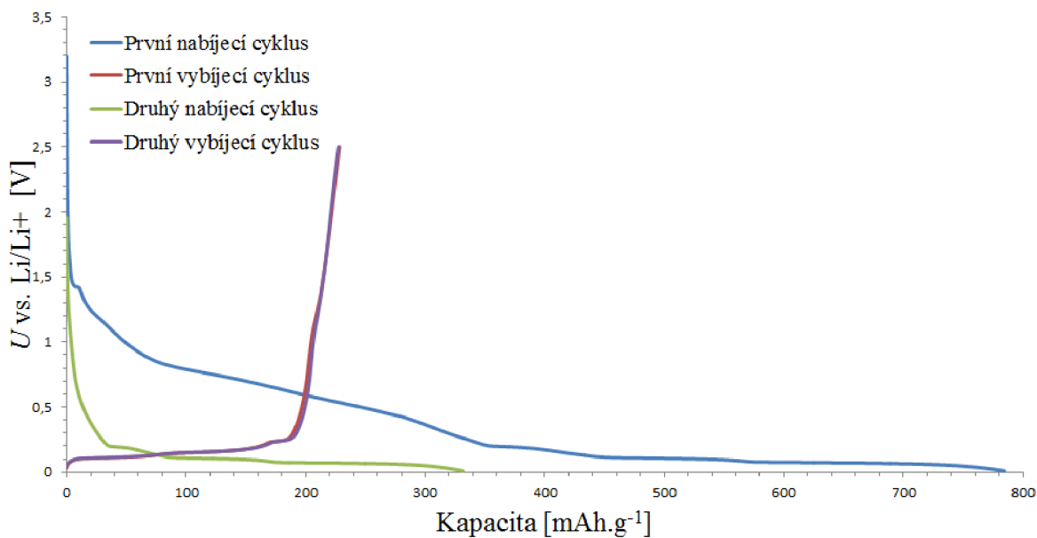
Obr. 57: První dva nabíjecí a vybíjecí cykly přírodního grafitu COND 5995 lisovaného tlakem 100 \text{ kg.cm}^{-2}
