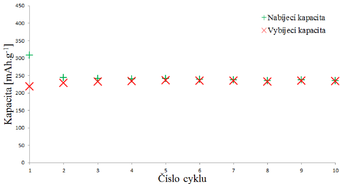
Obr. 49: Nabíjecí a vybíjecí kapacita každého cyklu přírodního grafitu 280 H lisovaného tlakem 2000 kg.cm -2
