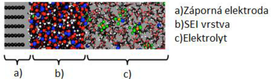
Obr. 3: SEI vrstva [13]
