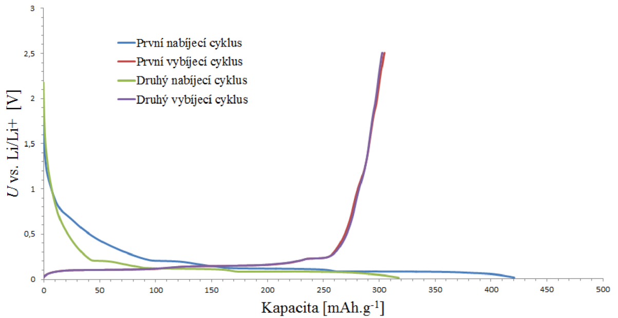
Obr. 45: První dva nabíjecí a vybíjecí cykly přírodního grafitu 280 H lisovaného tlakem 1000 \text{ kg.cm}^{-2}
