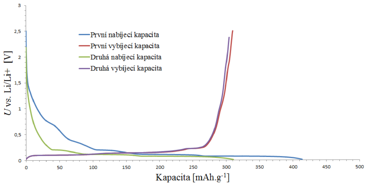
Obr. 39: První dva nabíjecí a vybíjecí cykly přírodního grafitu 280 H lisovaného tlakem 300 \text{ kg.cm}^{-2}
