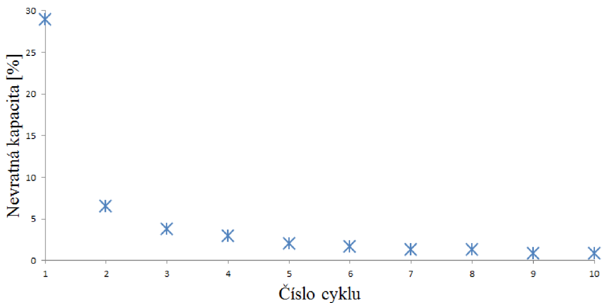
Obr. 50: Nevratná kapacita každého cyklu přírodního grafitu 280 H lisovaného tlakem 2000 kg.cm -2
