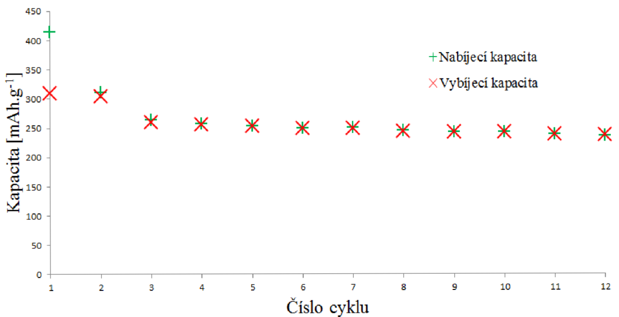
Obr. 40: Nabíjecí a vybíjecí kapacita každého cyklu přírodního grafitu 280 H lisovaného tlakem 300 \text{ kg.cm}^{-2}
