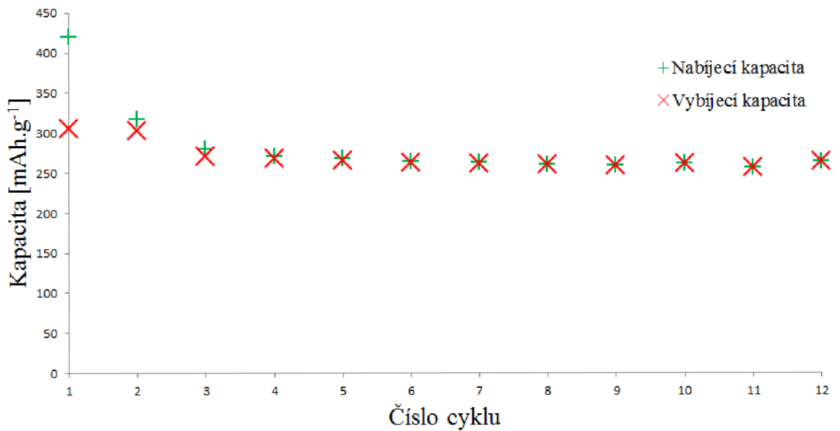
Obr. 46: Nabíjecí a vybíjecí kapacita každého cyklu přírodního grafitu 280 H lisovaného tlakem 1000 \text{ kg.cm}^{-2}
