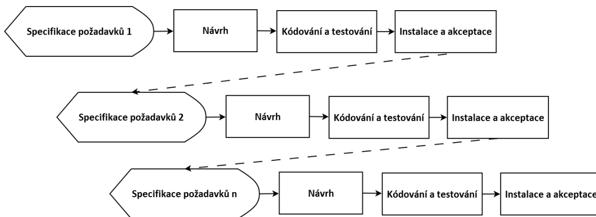
Obrázek 4 Evoluční model
