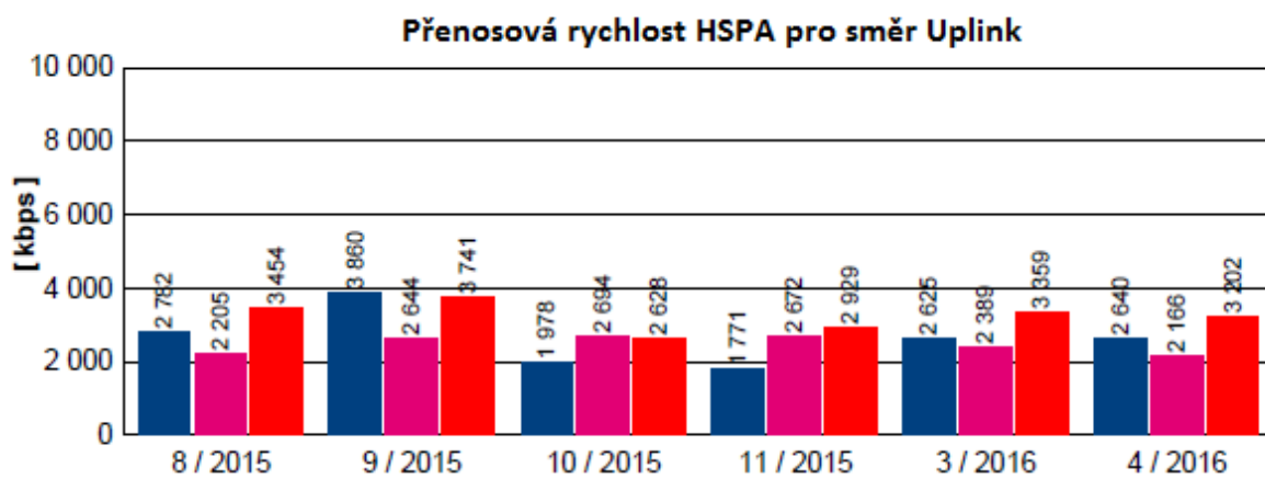
Obr. 6.3: Přenosová rychlost technologie HSPA pro směr Uplink na Praze 5 [31].
