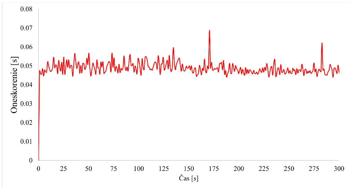
Obr. 6.10: Priebeh oneskorenia so spusteným NewShrew útokom s interburst periódou 1800 ms a burst periódou 50 ms počas tridsiatich minút s aplikovaným IDS/IPS na filtračnom serveri.
