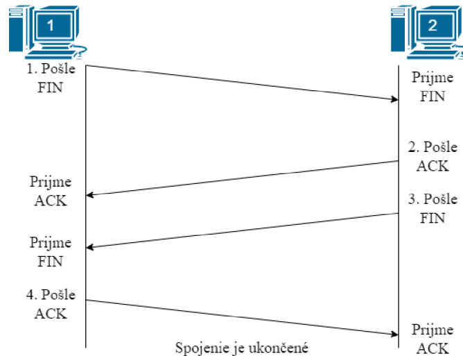
Obr. 1.4: Ukončenie TCP spojenia.
