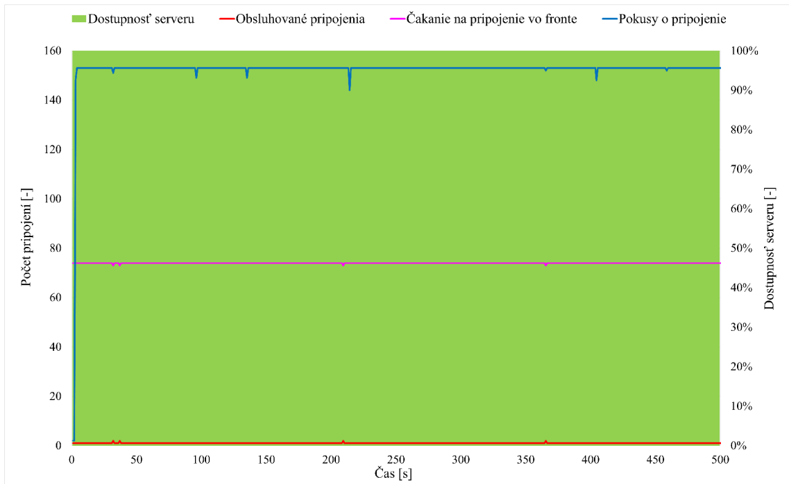
Obr. 7.7: Zobrazenie spracovávania požiadaviek vo fronte pomocou modulu MPM event na webovom servery.
