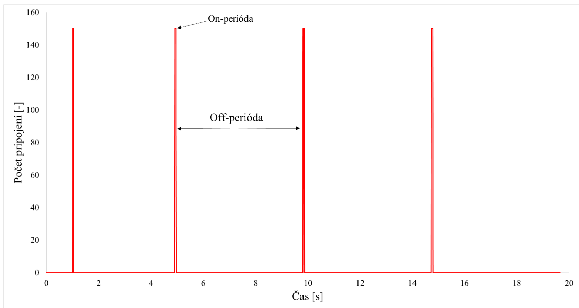
Obr. 7.1: Priebeh LoRDAS útoku s off periódou 4.85 sekundy a 150 keep-alive požiadaviek v on-periódou.
