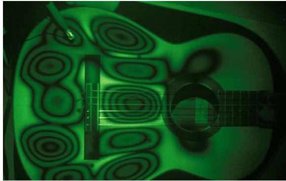
Obr. č. 33 – Metoda holografické interferometrie (compadre.org).
