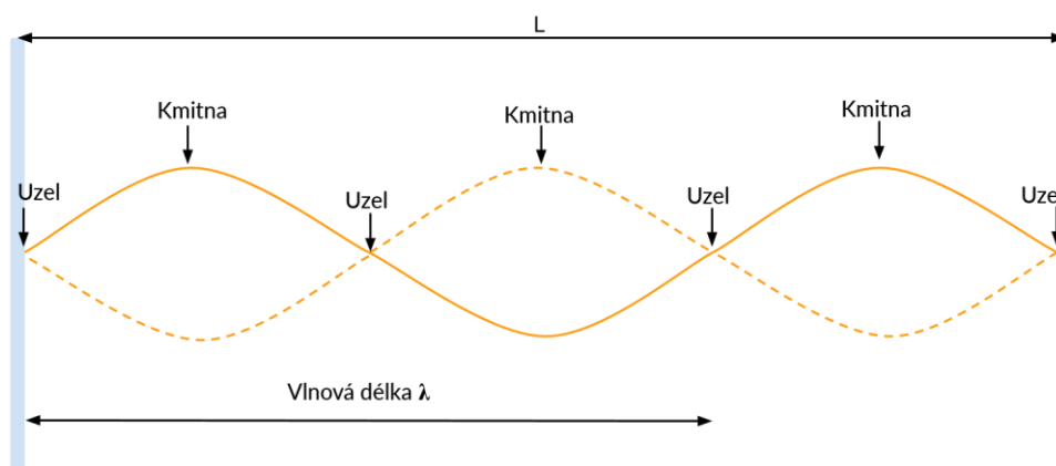
Obr. č. 30 – Stojaté vlnění ( cdn.kastatic.org ).
