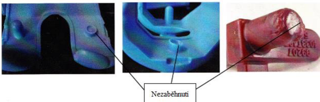
Obr. 20 Nezaběhnutí vosku do matečné formy [37]
