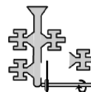
CH) Odřezání odlitků od vtokového systému
