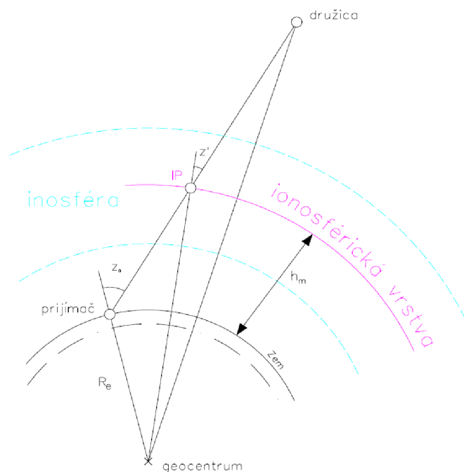
Obr. 10: Schéma ionoférickej vrstvy, upravené [21]
