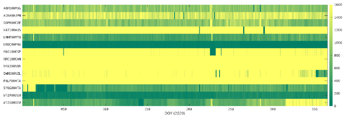
Obr. 24: Počet cycle slips pre systém GLONASS
