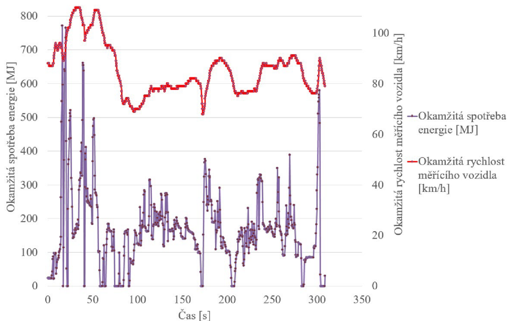
Obr. 24: Dálnice D10 pravý provizorní pruh (směr Praha)
