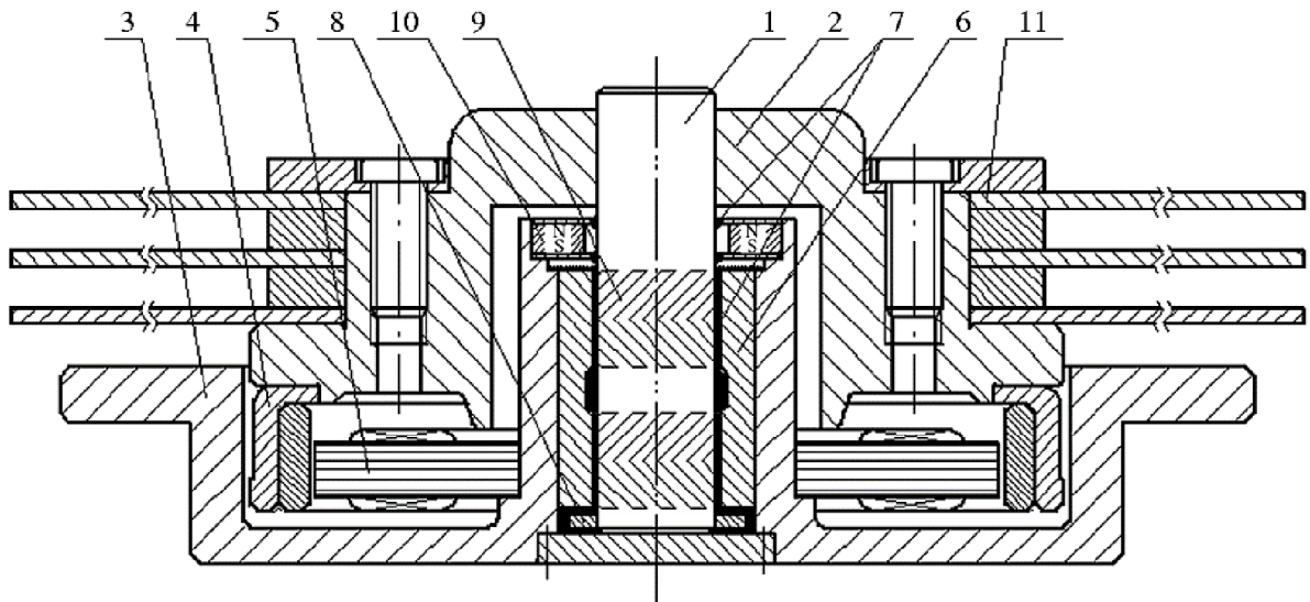
1 - hřídel, 2 - náboj, 3 - stator, 4 - rotor, 5 - jádro statoru, 6 - pouzdro kluzného ložiska, 7 - magnetická kapalina, 8 - přítlačná deska, 9 - drážka, 10 - ucpávka s magnetickou kapalinou, 11 - magnetický disk
