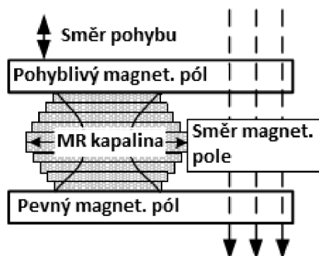
Obr. 8 Tlakový mód MR kapaliny [3]
