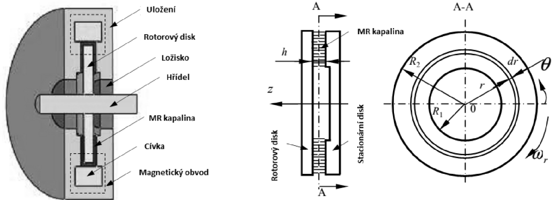
Obr. 13 Brzda s magnetoreologickou kapalinou [7]
