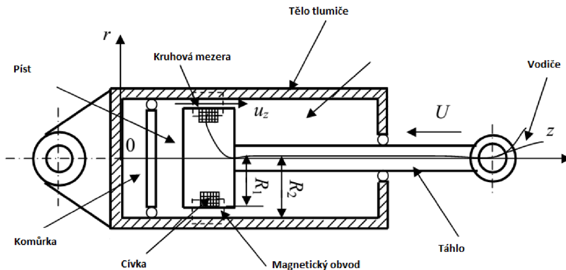
Obr. 12 Schématický náčrt magnetoreologického tlumiče [8]
