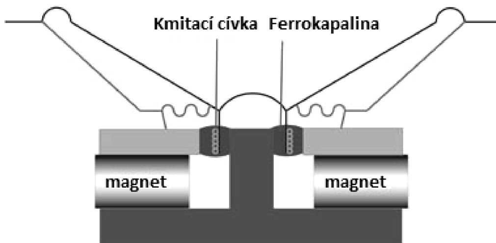
Obr. 15 Reproduktor využívající ferrokapalinu [17]
