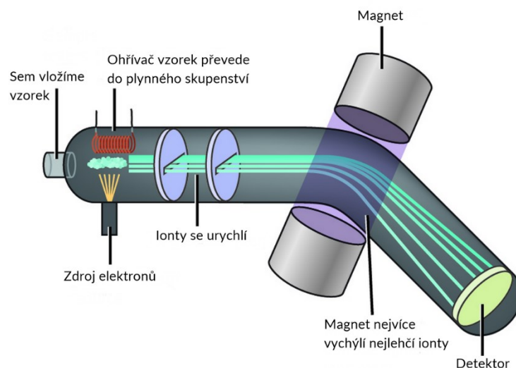
Obr. 10: Znárodnění základního mechanismu hmotnostního spektrometru.
