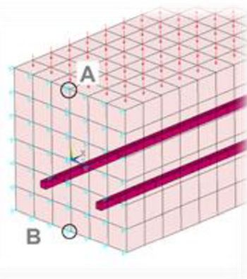
Obr. 2.10 Analyzované miesta v strednom priereze
