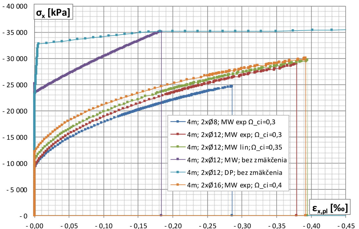
Graf 2.2 Závislosť normálového napätia \sigma_x v horných vláknach betónu na pomernej deformácii \epsilon_{x,pl} (výstupy z bodu A obrázku 2.10)
