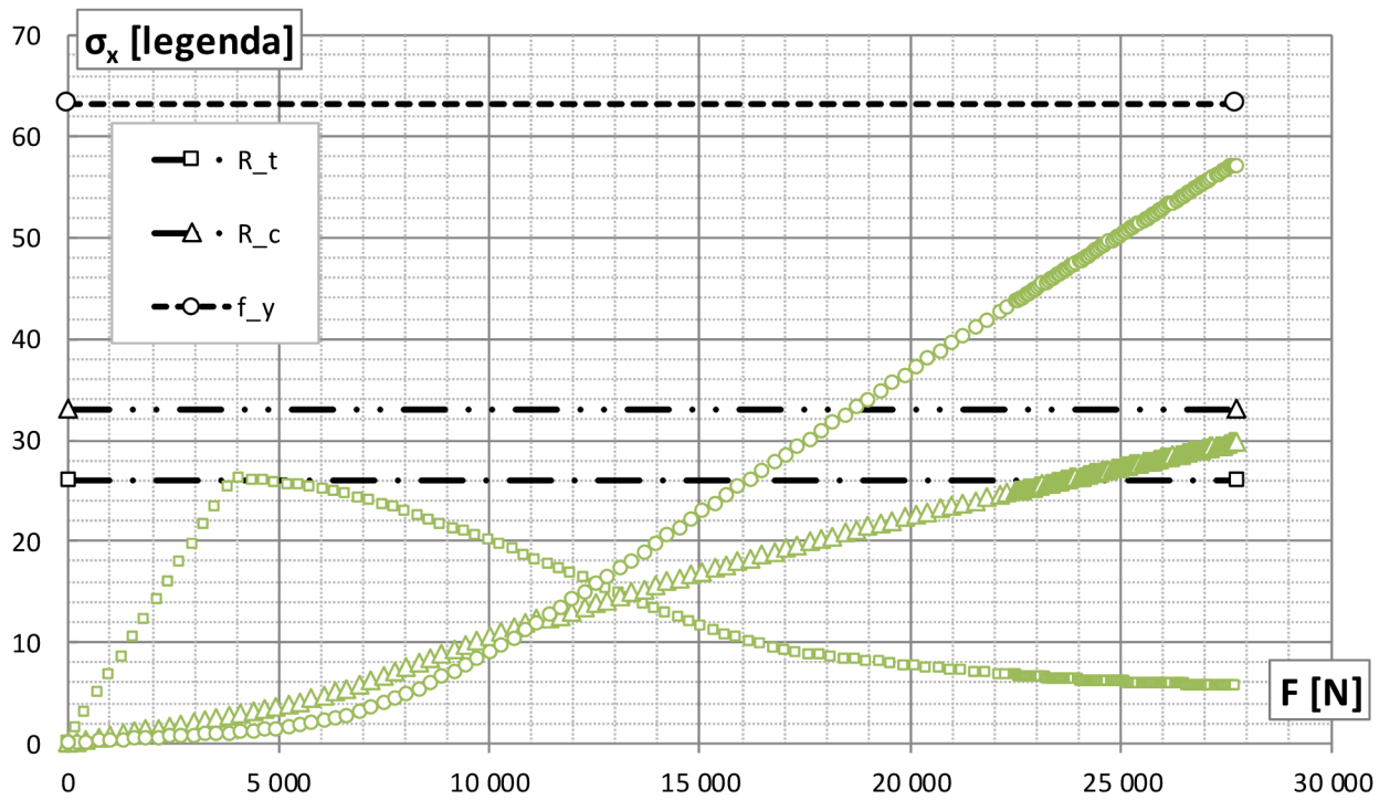
Graf 2.12 Závislosť napätí na zaťažení F v sledovaných bodoch konštrukcie pre prípad 9
