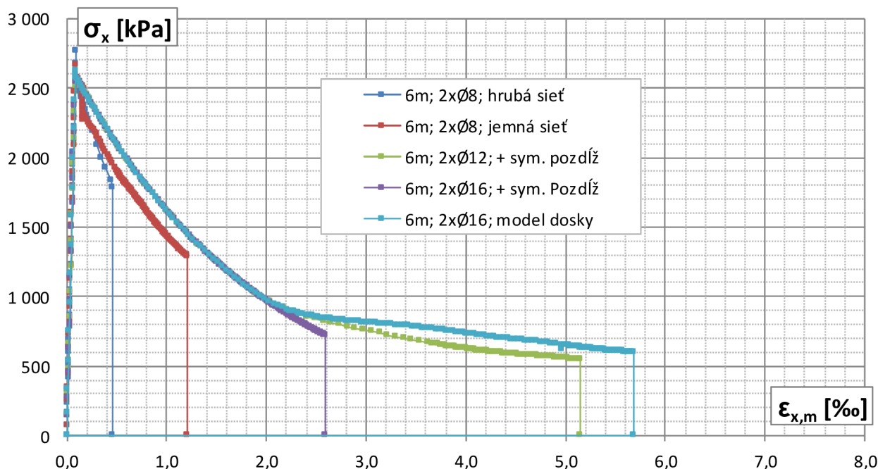
Graf 2.7 Závislosť normálového napätia \sigma_x na pomernej deformácii \epsilon_{x,m} (v bode B)
