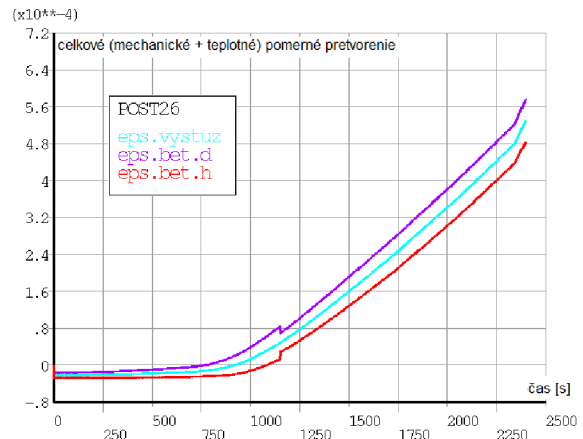
Obr. 3.50 Celkové pomerné deformácie vo výstuži a betóne
