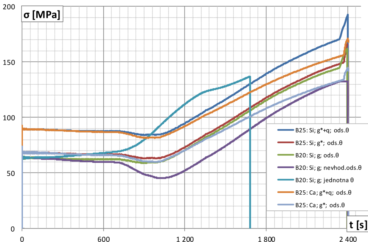
Graf 3.33 Časový priebek pozdĺžneho napätia v bode v spodnej časti nosníka
