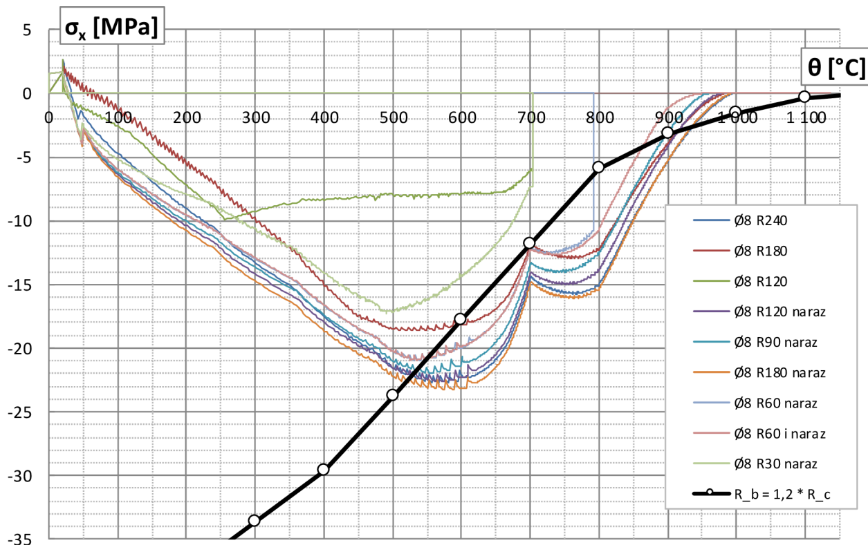
Graf 2.39 Priebeh napätia v spodných vláknoch dosky v strede rozpätia v závislosti na ich teplote
