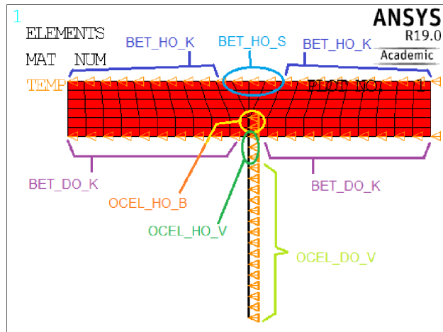
Obr. 3.25 Aplikovanie zaťaženia
