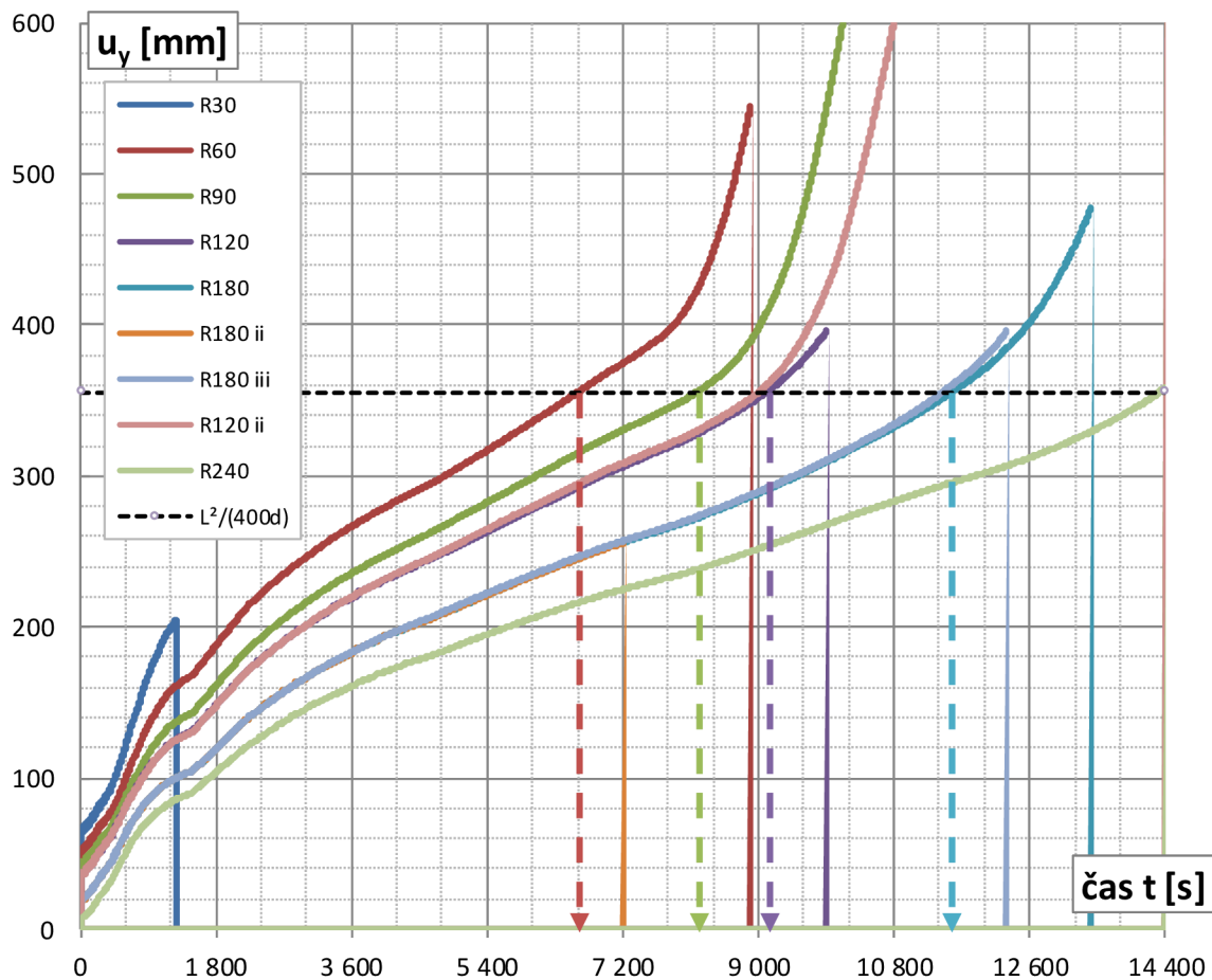
Graf 2.22 Priebeh priehybu v strede rozpätia dosky v závislosti na čase t
