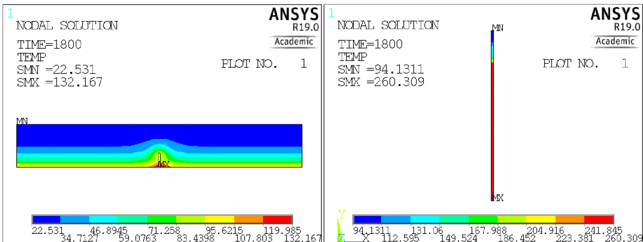
Obr. 3.26 Detail teplotného poľa v čase 30 min: vľavo dosky; vpravo ocelového nosníka
