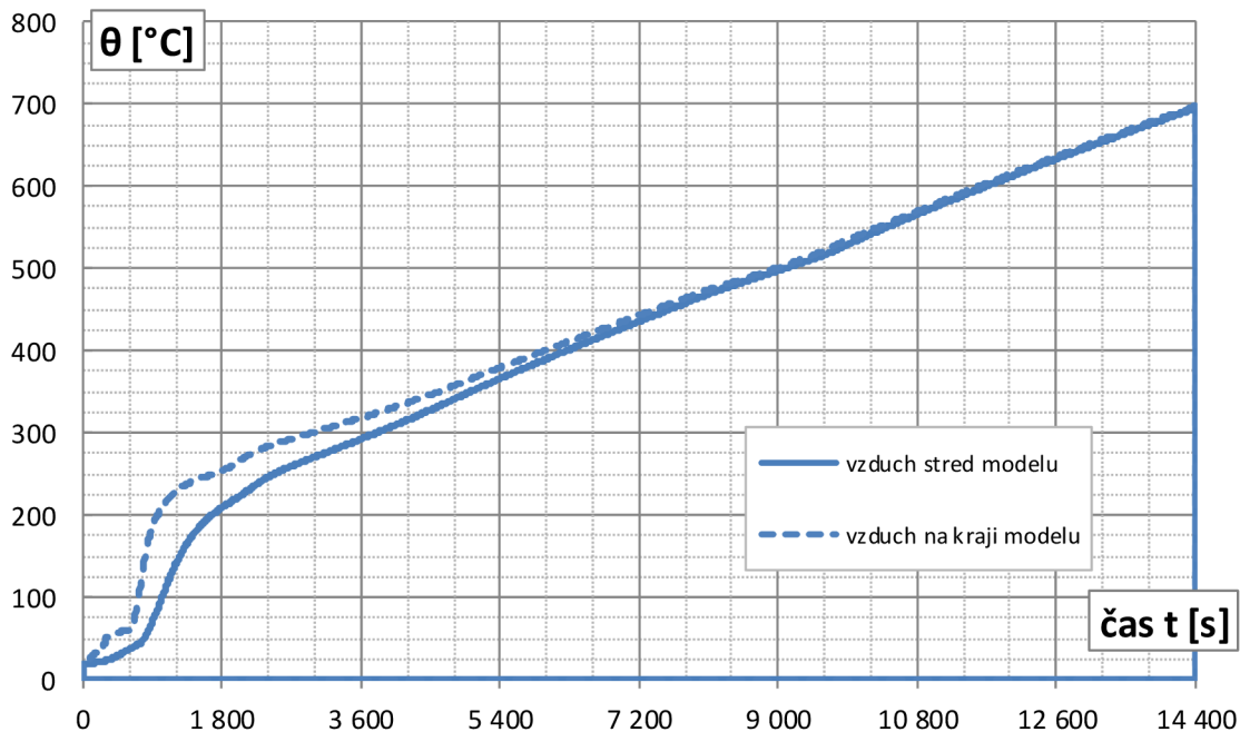
Graf 3.11 Priebeh teplôt v bodoch v strede výšky vzduchovej vrstvy v dvoch rôznych miestach pre prípad s označením " \varepsilon = 1 všade; veľký"
