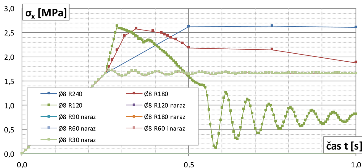
Graf 2.40 Priebeh normálového napätia v spodných vláknoch dosky v priebehu 1. sekundy analýz
