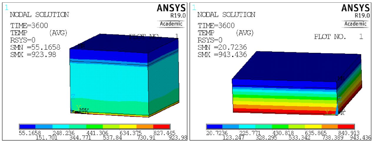
Obr. 3.16 Porovnanie rozloženia teplotného poľa v čase 60 min pre model "stredný" (50 cm hrana) a hodnotou \varepsilon = 1 (modrá krivka na grafoch) - vľavo; vpravo pri zanedbaní radiácie
