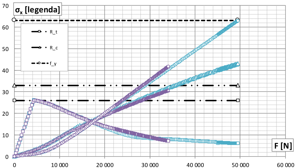
Graf 2.13 Závislosť napätí na zaťažení F v sledovaných bodoch konštrukcie pre prípady 10 a 11
