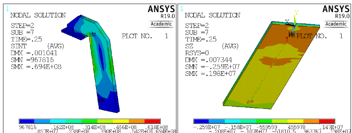
Obr. 3.43 Čas T = 0,25 s: vľavo intenzita porovnávacieho napätia na závesnej pätky [Pa]; vpravo pozdĺžne napätie v betónovej doske [Pa]
