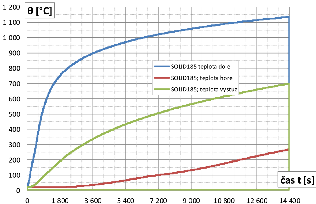
Graf 2.20 Priebehy teplôt v čase v sledovaných miestach konštrukcie
