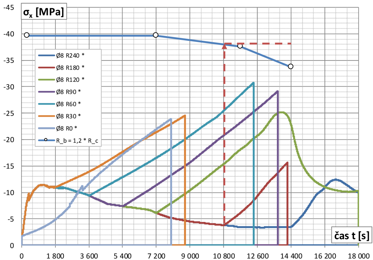
Graf 2.45 Časový priebeh napätia \sigma_x v horných vláknach dosky v strede rozpätia
