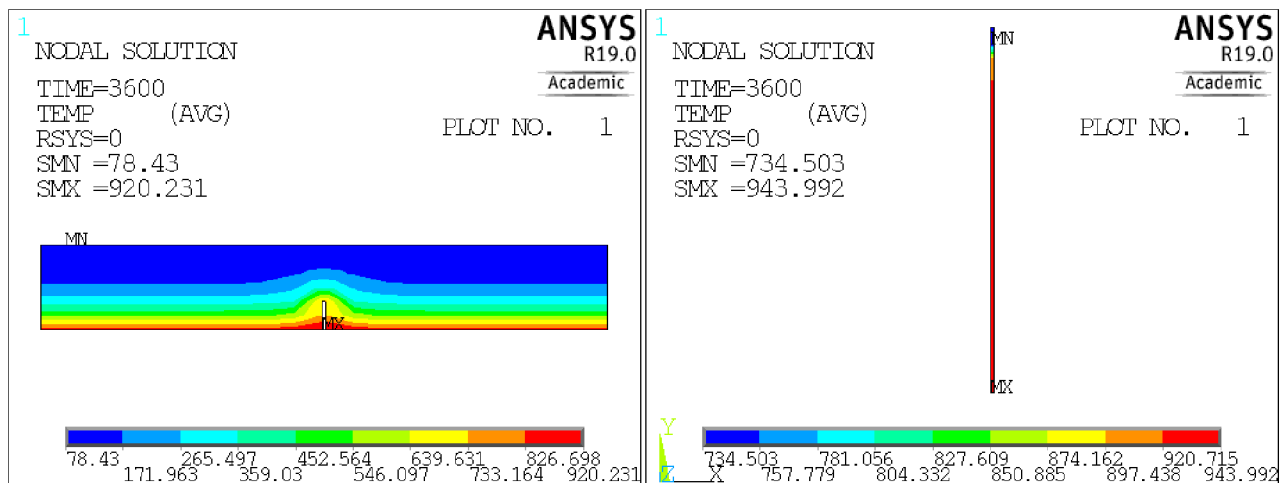
Obr. 3.29 Detail teplotného poľa v čase 60 min: vľavo dosky; vpravo ocelového nosníka
