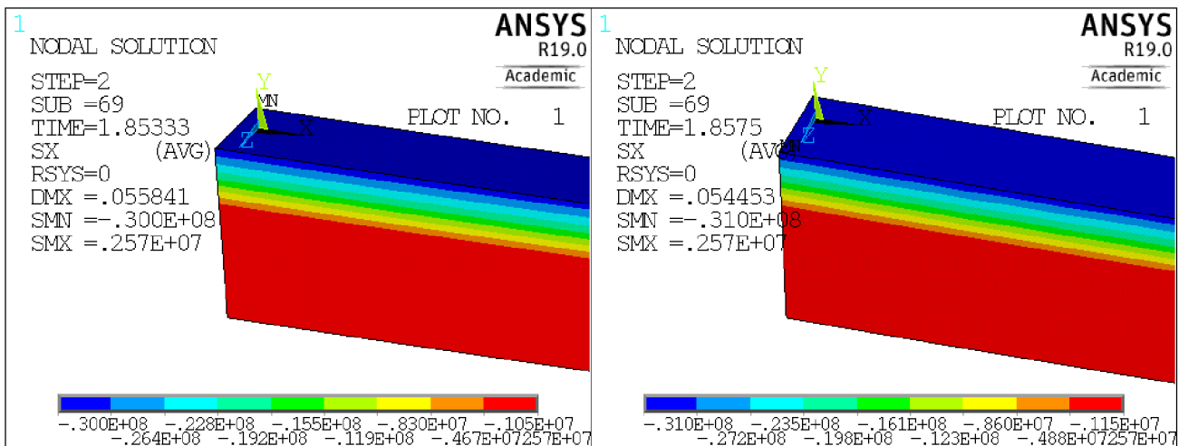
Obr. 2.18 Normálové napätia \sigma_x [Pa]: vľavo model bez strmienkov, vpravo osovo po 75 mm
