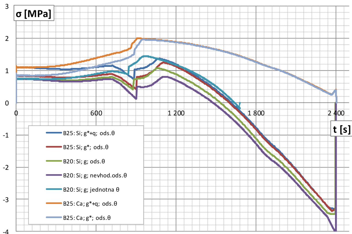
Graf 3.29 Časový priebeh pozdĺžneho napätia na spodnom povrchu betónovej dosky
