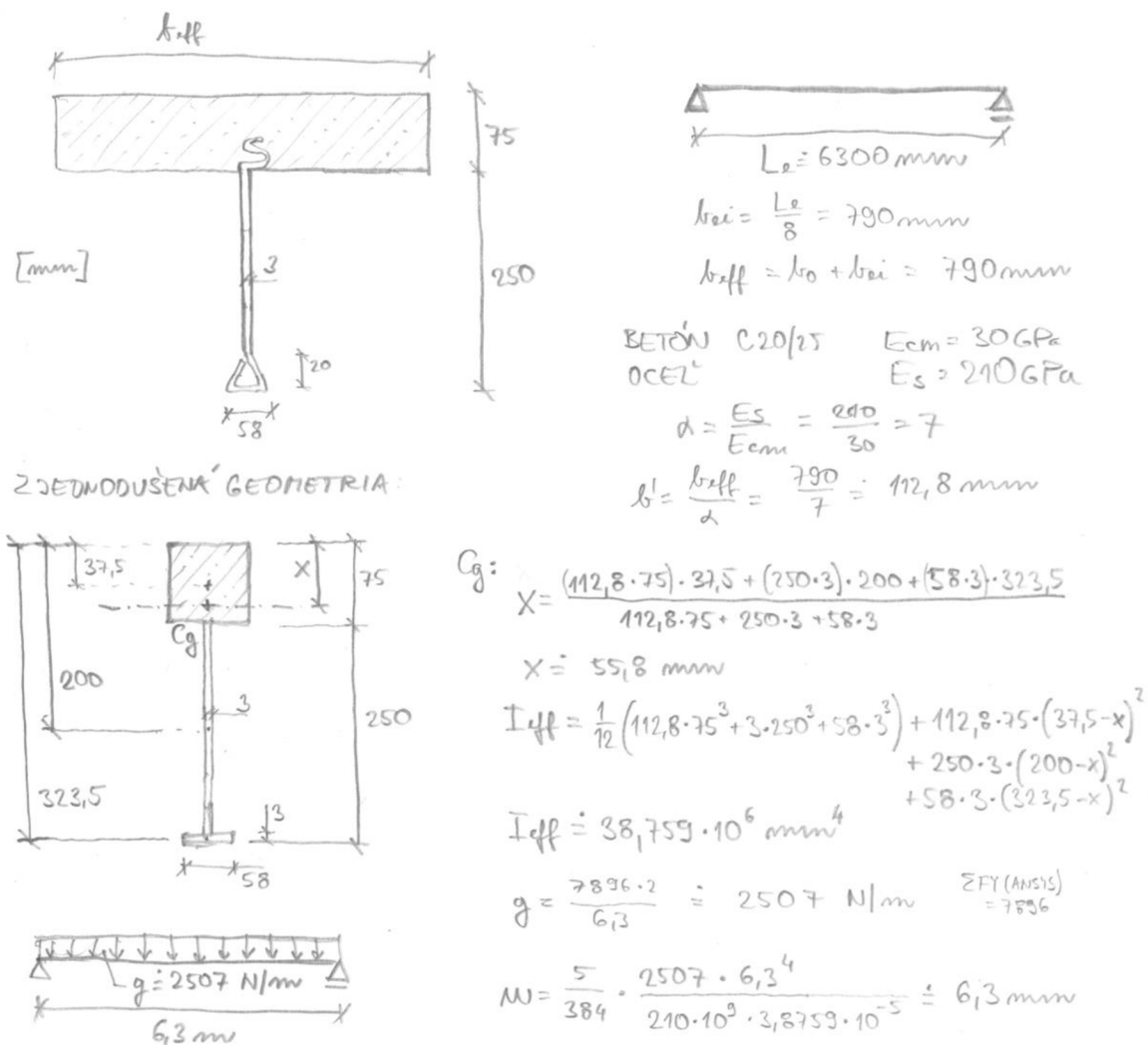
Obr. 7.1 Orientačné určenie priehybu
