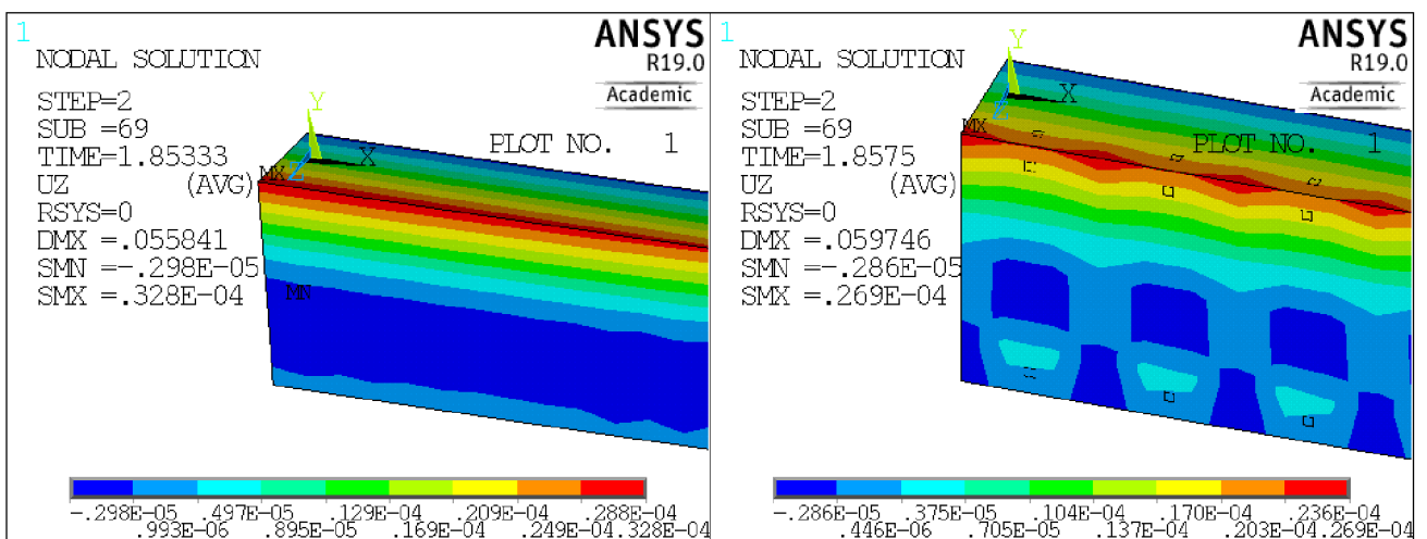
Obr. 2.19 Priečny posun u_z [m]: vľavo model bez strmienkov, vpravo osovo po 75 mm
