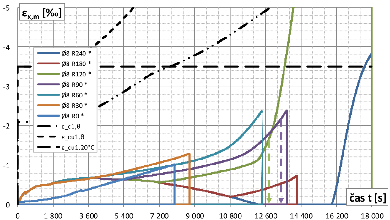
Graf 2.46 Časový priebeh pomernej mechanickej deformácie v horných vláknach dosky v strede rozpätia
