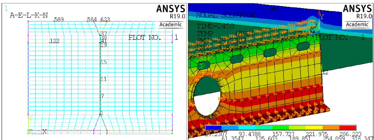
Obr. 3.34 Vľavo: doplnenie referenčných bodov pre sledovanie priebehu teploty na 2D modeli; vpravo: výsledok teplotného poľa v čase t = 2400 s pri definovaní teploty bodom na nosníku po líniiach
