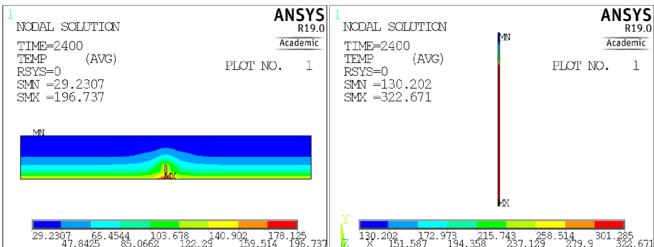
Obr. 3.27 Detail teplotného poľa v čase 40 min: vľavo dosky; vpravo ocelového nosníka
