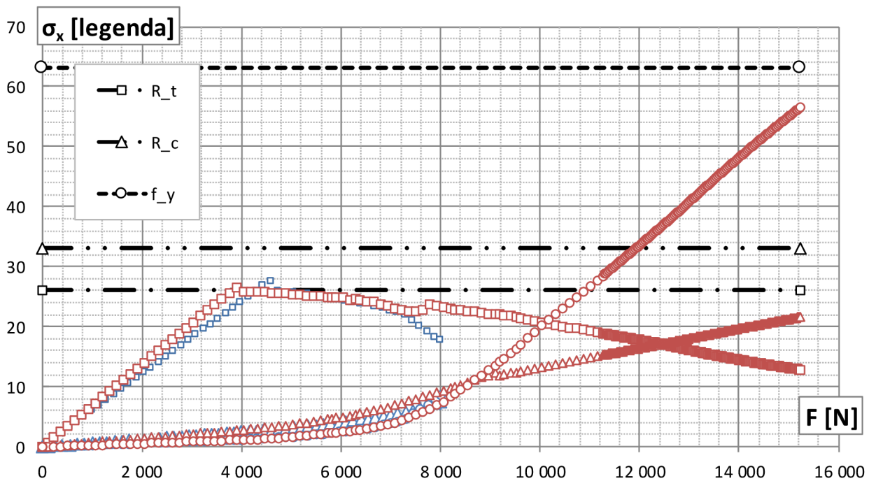
Graf 2.11 Závislosť napätí na zaťažení F v sledovaných bodoch konštrukcie pre prípady 7 8
