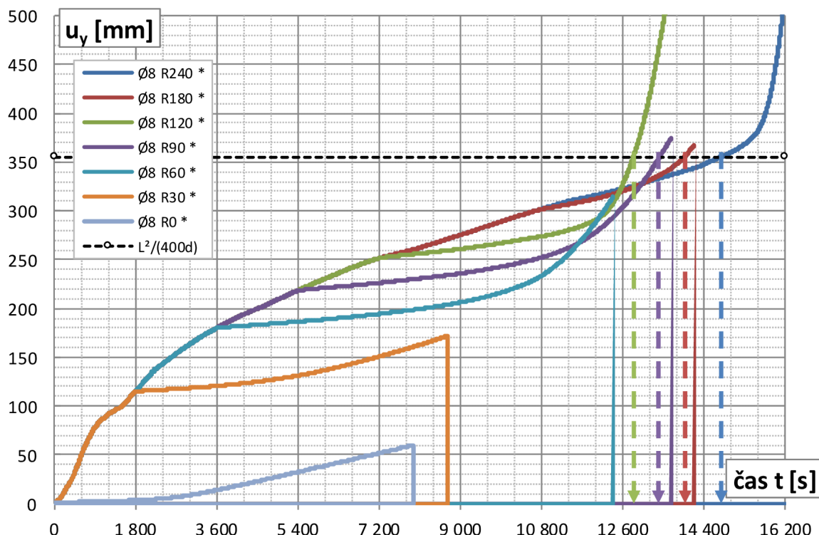
Graf 2.41 Časový priebeh zvislého prihybu v strede rozpätia dosky
