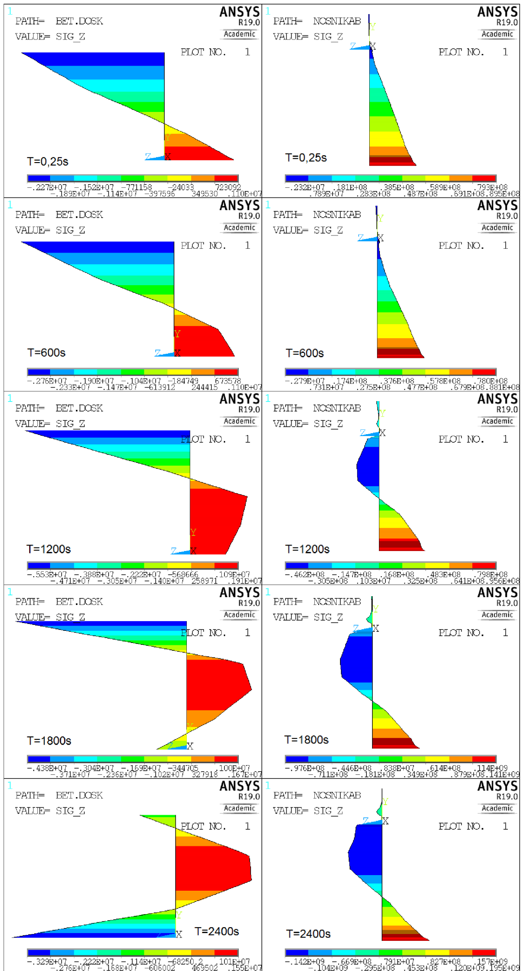
Obr. 3.45 Priebek pozdĺžnych napätí [Pa] v rezoch v strede rozpätia v rôznych časoch T pre prípad označený v grafických legendách ako "B25: Si; g^*+q ; ods. \theta "
