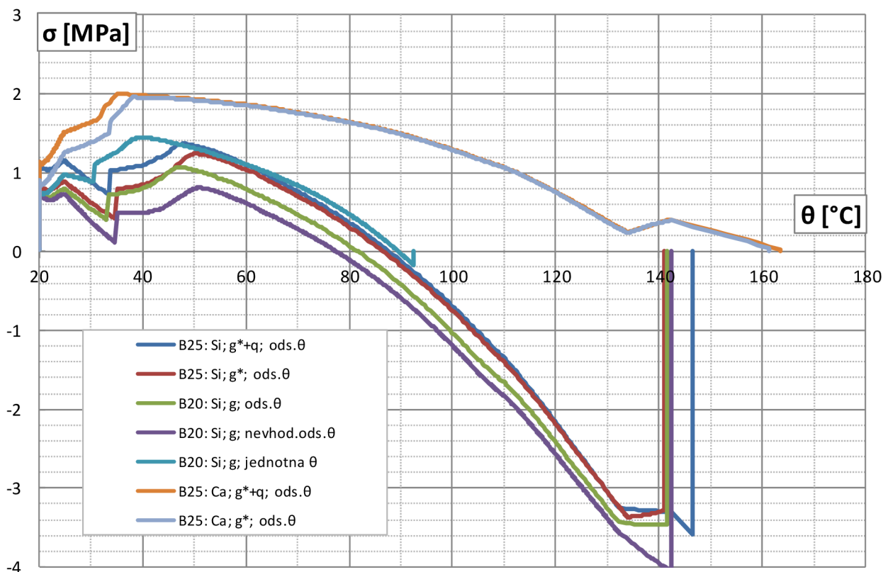
Graf 3.28 Priebeh normálového (pozdĺžneho) napätia vo vybranom bode na spodnom (ohrievanom) povrchu betónovej dosky v závislosti na teplote v tomto bode.
