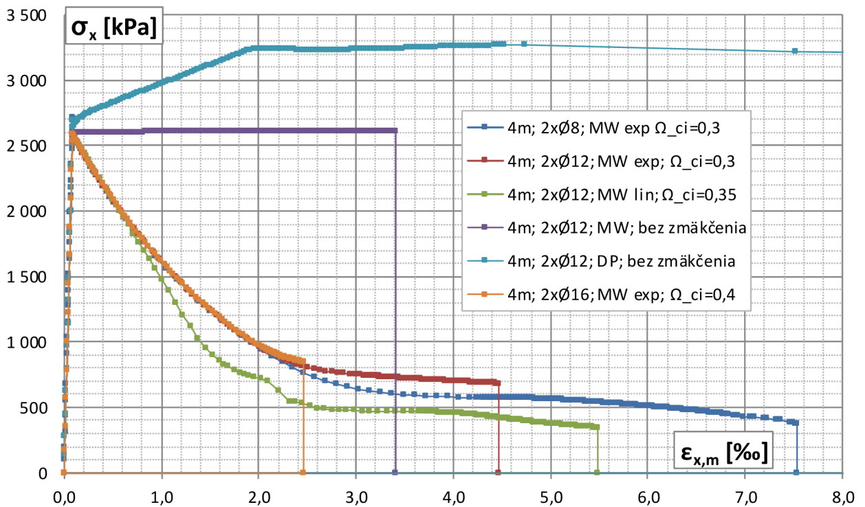
Graf 2.1 Závislosť normálového napätia \sigma_x v spodných vláknach betónu na pomernej deformácii \epsilon_{x,m} (výstupy z bodu B obrázku 2.10)
