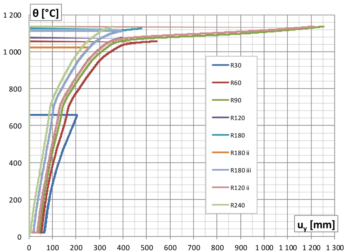
Graf 2.23 Priebeh teploty na spodnej hrane dosky v závislosti na zvislom priehybe v strede rozpätia
