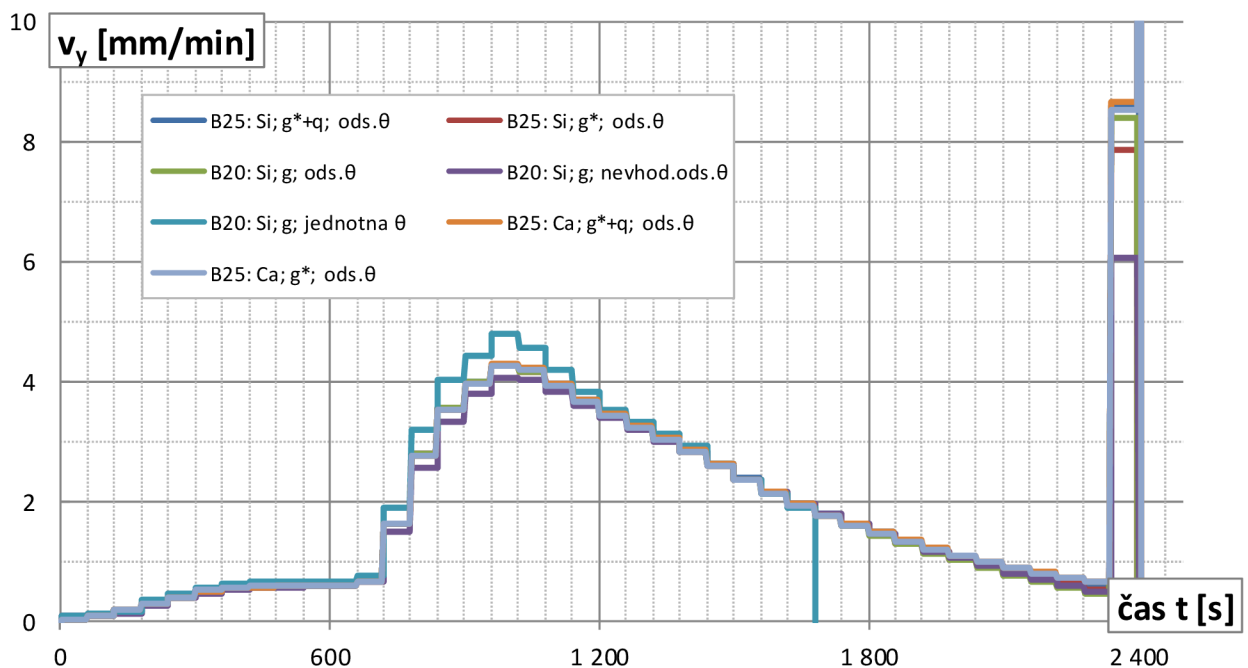
Graf 3.25 Časový priebeh rýchlosti posunu bodu na spodnej časti nosníka
