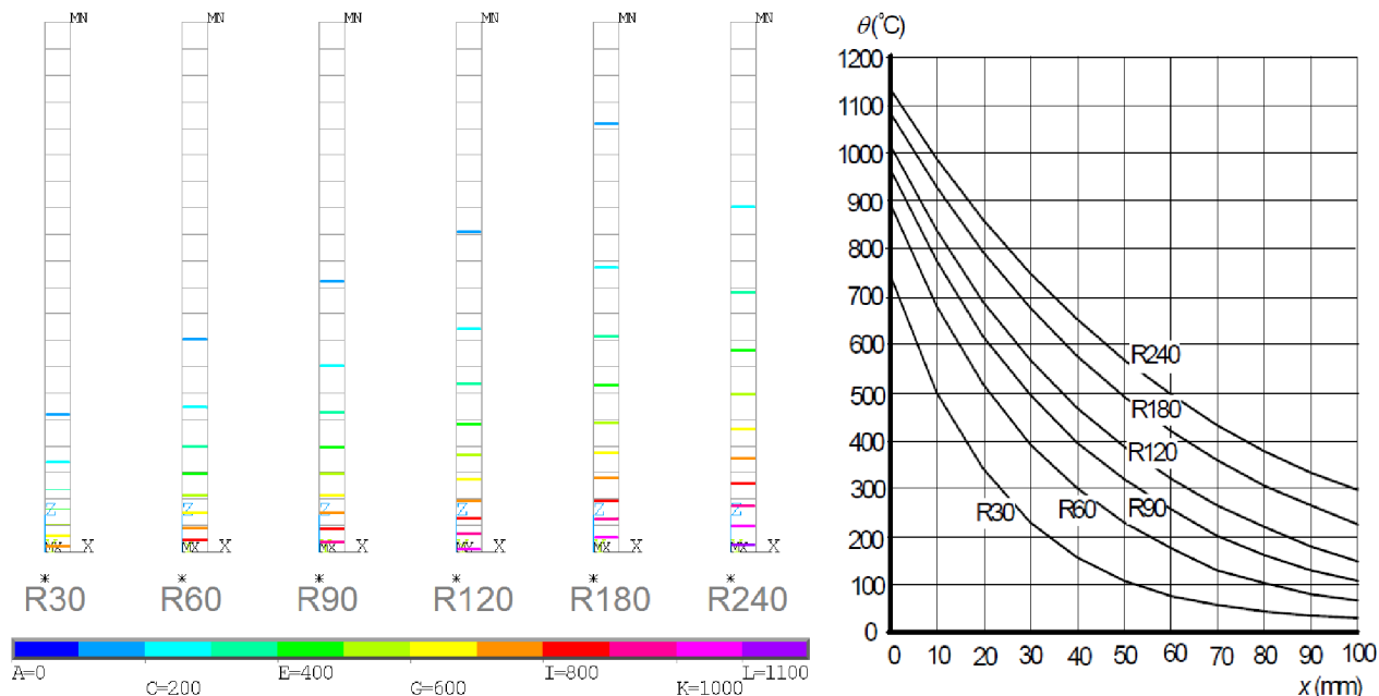
Obr. 2.30 Teplotné profily pre dosky hrúbky 200 mm: vľavo izotermi získané výpočtom v prostredí ANSYS; vpravo podľa prílohy A literatúry (3)
