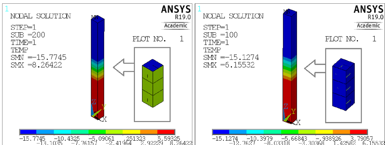
Obr. 3.13 Vľavo: priebeh teplôt pri hodnote \varepsilon = 0 (resp. 1E-16 ) pre elementy na plášti hranola; vpravo: priebeh teplôt pri hodnote \varepsilon = 1 pre elementy na plášti hranola
