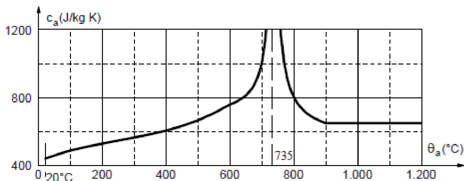
Obr. 2.26 Merná tepelná kapacita oceli c_a podľa (8)
