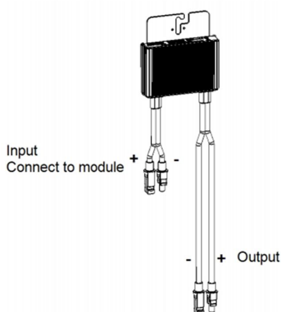
Obr. 11: Schéma optimizéru [12]
