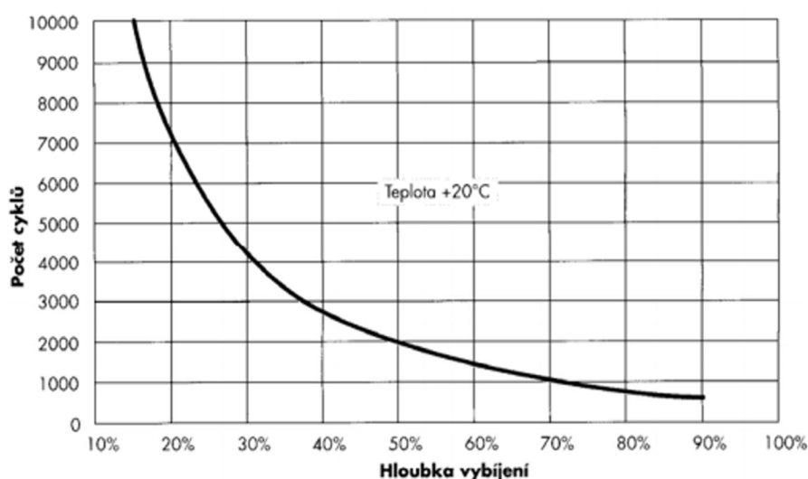
Obr. 5: Počet cyklů závislých na hloubce vybití u NiCd baterií [25]
