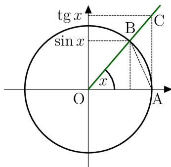
Obrázek 4.1: Nerovnost \frac{1}{2} \cdot \sin x < \frac{1}{2} \cdot x < \frac{1}{2} \cdot \operatorname{tg} x na jednotkové kružnici.
