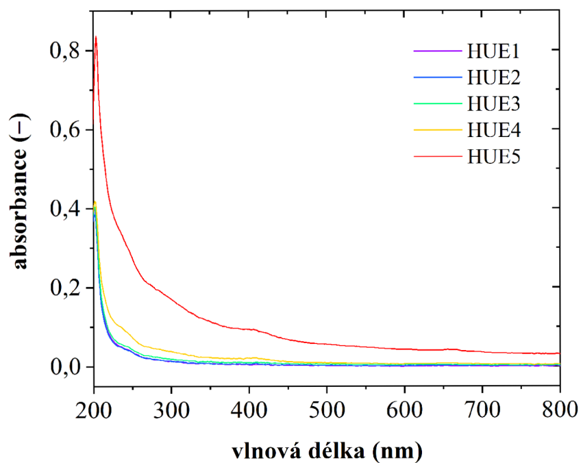
Obr. 24: UV/Vis spektra TLC frakcí HU izolovaného z alginitu
