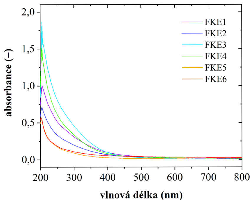
Obr. 23: UV/Vis spektra TLC frakcí FK izolované z alginitu
