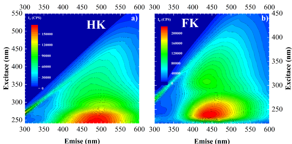
Obr. 12: Excitačně-emisní spektra izolovaných HL a) Alginit HK b) Alginit FK
