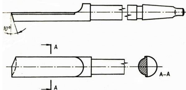
Obr. 1.7 Dělový vrták [9].
