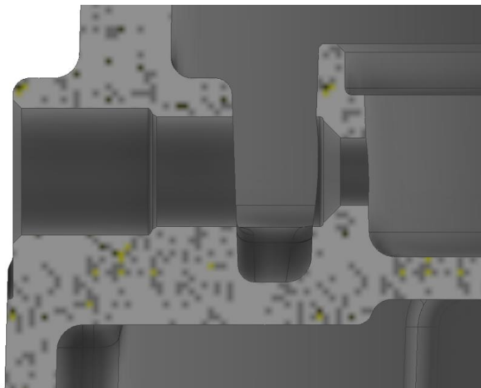
Obr. 4.1 Detail geometrie díry zamýšlené k vyvrtání sdruženým nástrojem.
